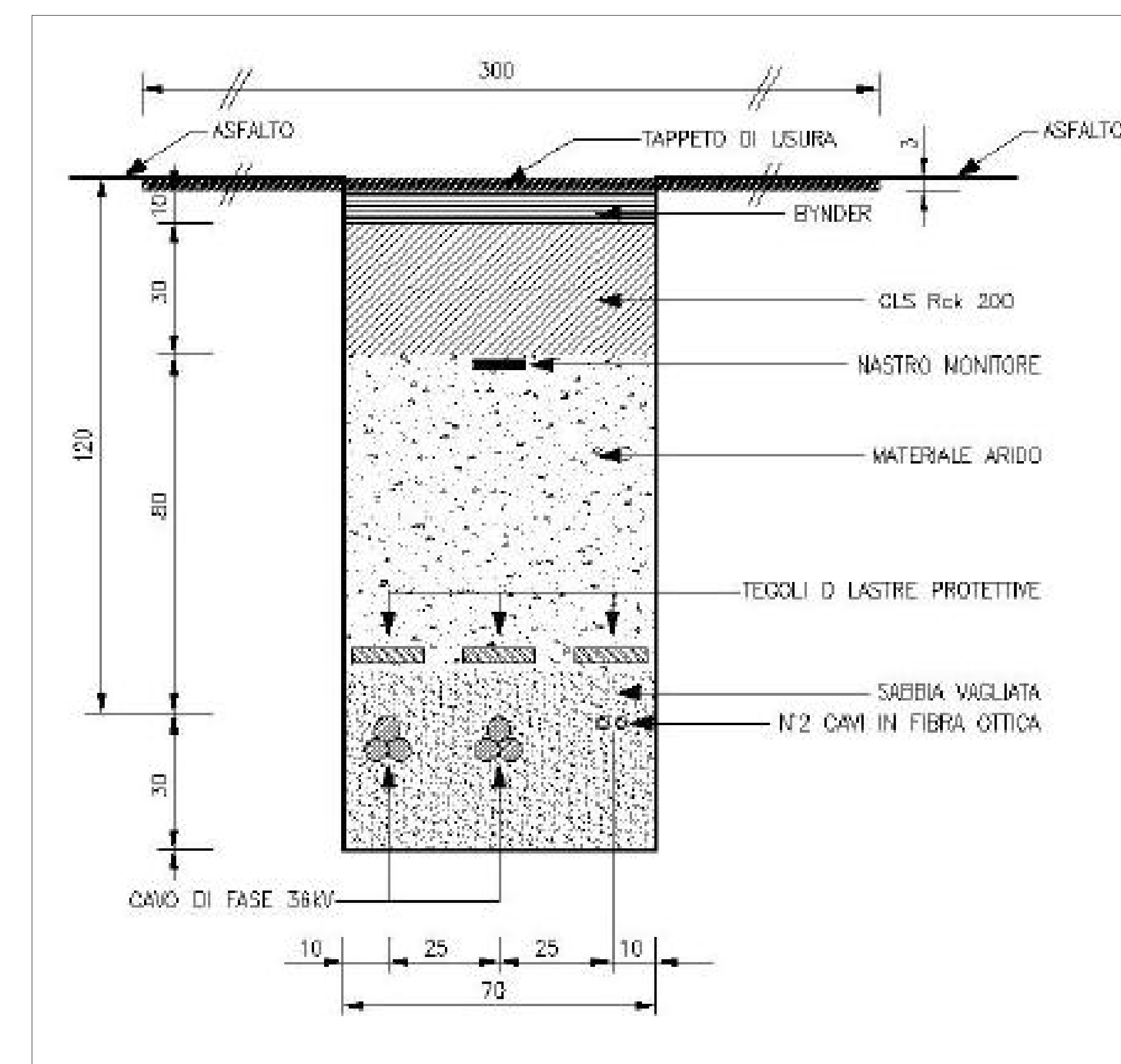
SCHEMA TIPO PARTICOLARE COSTRUTTIVO CAVIDOTTO INTERRATO AT
