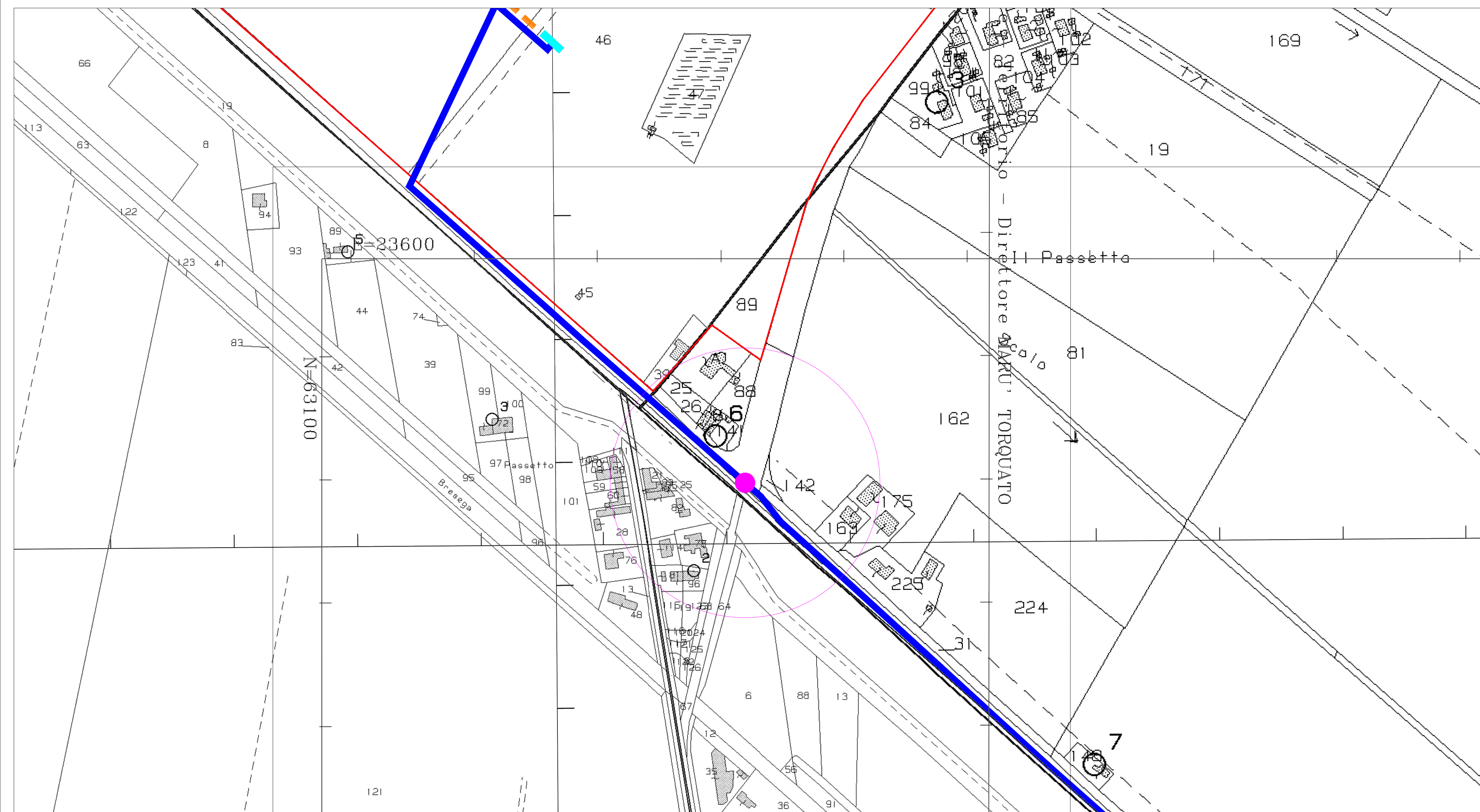
PARTICOLARE DELLO STATO ATTUALE SU CATASTALE CON INDICAZIONE DELLO SCAVO PER CAVIDOTTO INTERRATO
