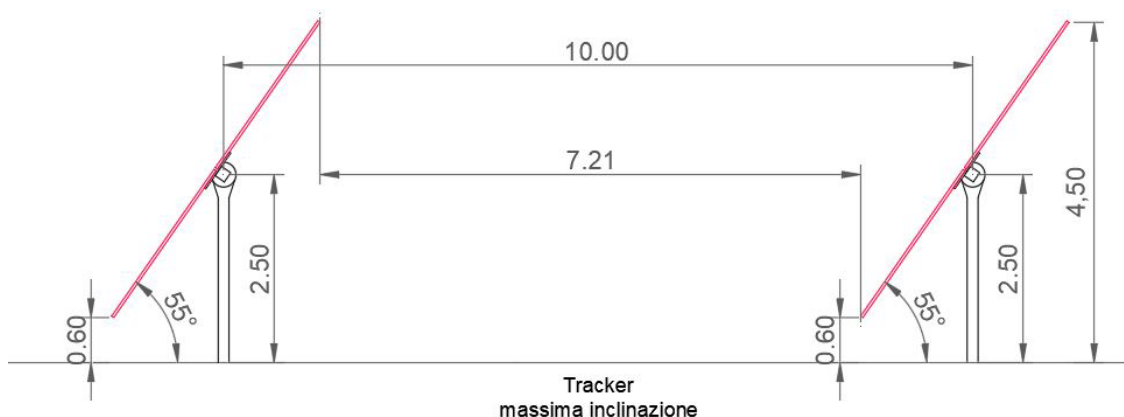
Figura 4 - particolari tracker
