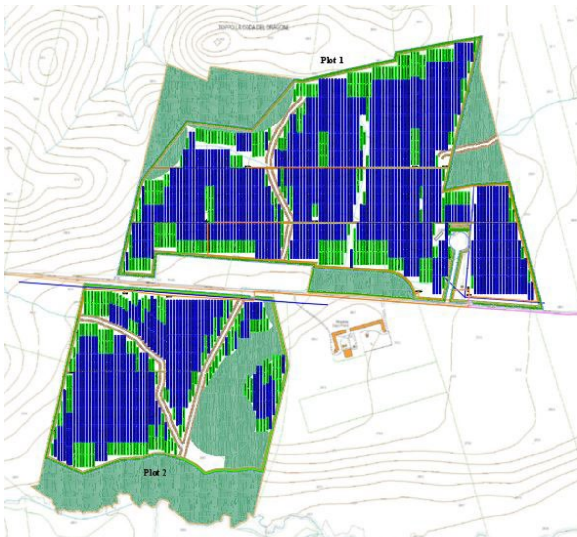
Figura 3 - Layout di progetto su CTR
