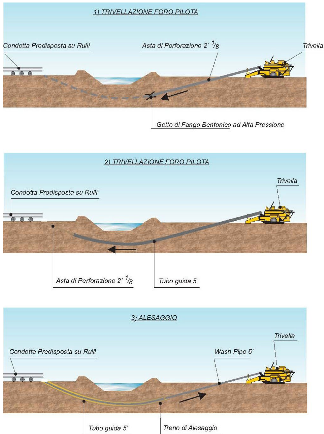
Figura 7 - trivellazione toc
