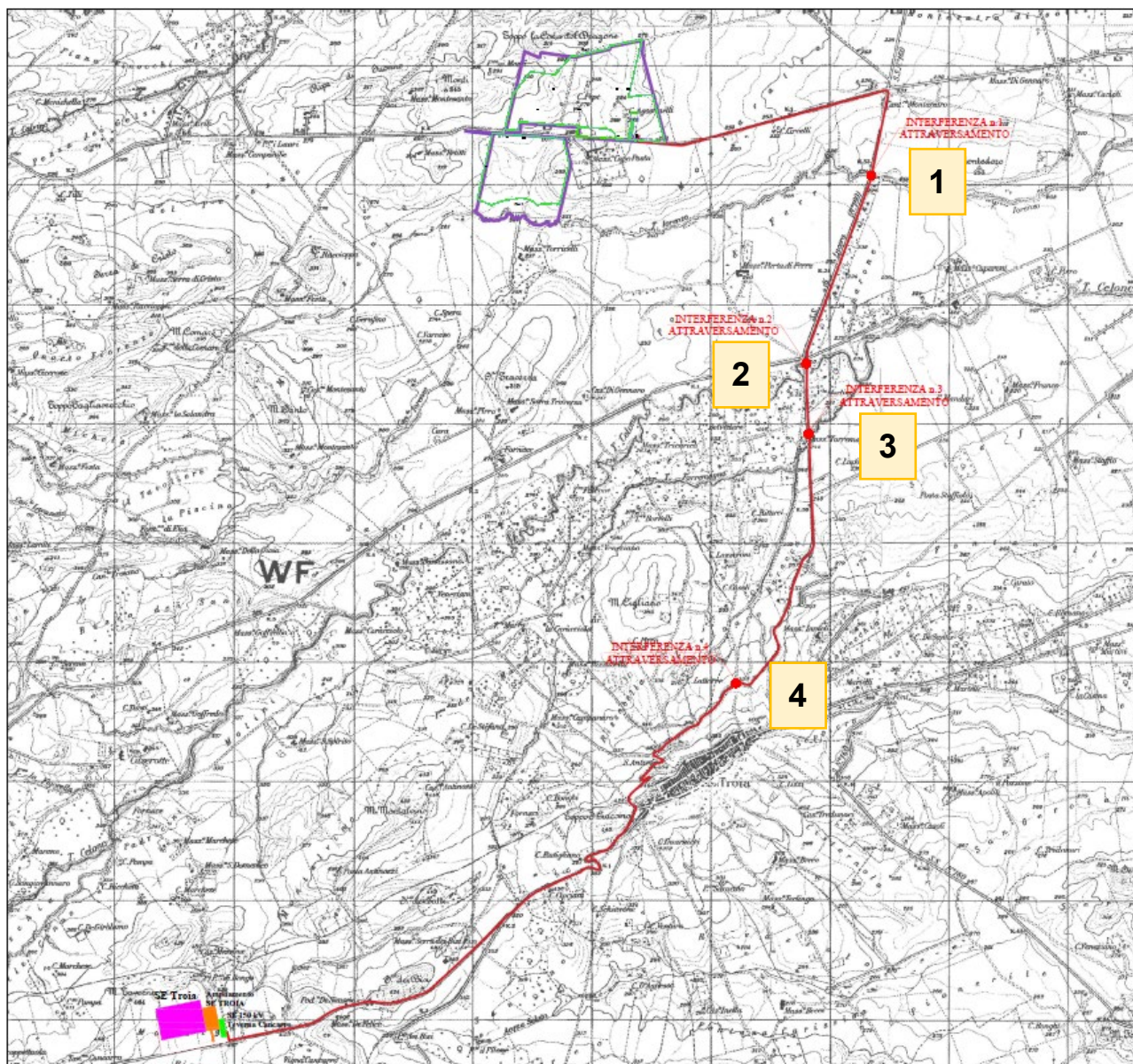
Figura 1 - Inquadramento planimetrico delle interferenze principali
