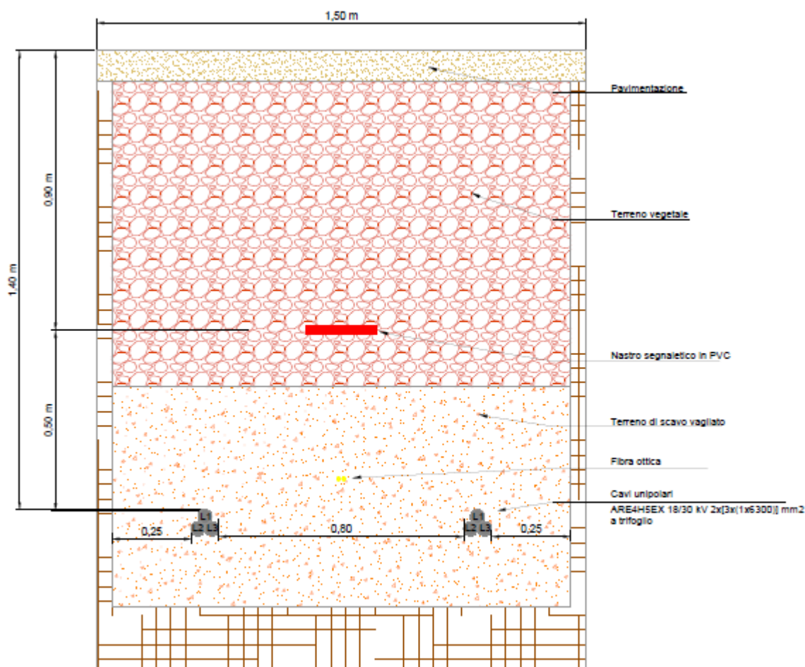
Figura 4 - particolare posa dorsali 36 kV
