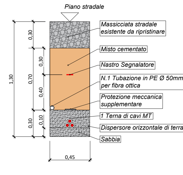
SEZIONE DI POSA "1EM" STRADA MASSICCIATA ESISTENTE
