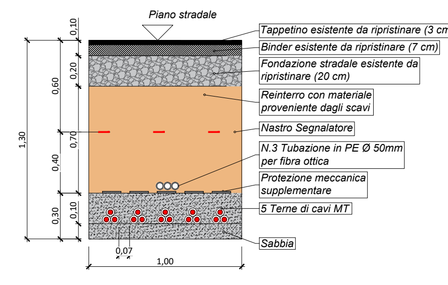
SEZIONE DI POSA "5AN" STRADA ASFALTATA ESISTENTE
