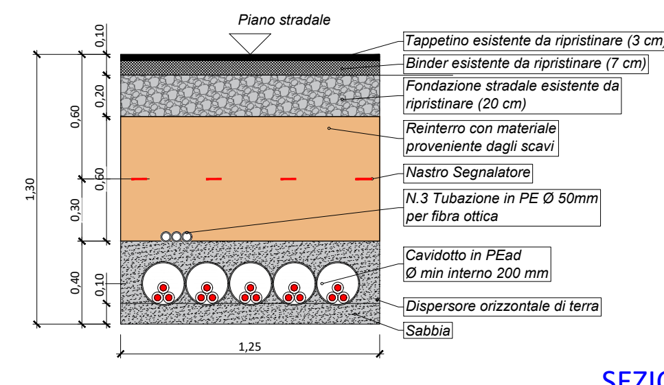
SEZIONE DI POSA "5AN" STRADA ASFALTATA ESISTENTE
