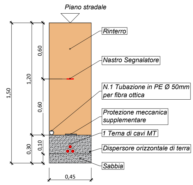
SEZIONE DI POSA "1TM" "1T TERRENO O BANCHINA STRADALE"
