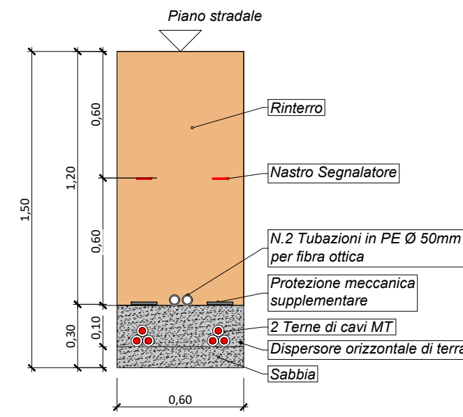
SEZIONE DI POSA "2TM" "2T TERRENO O BANCHINA STRADALE"
