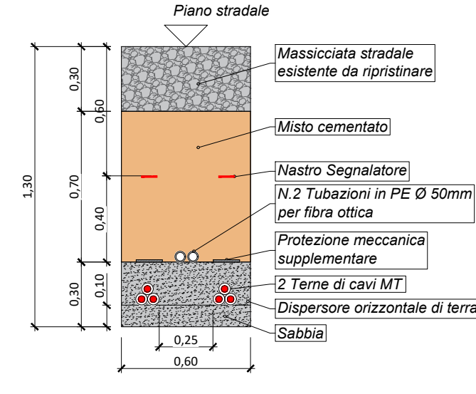
SEZIONE DI POSA "3AM" STRADA ASFALTATA ESISTENTE
