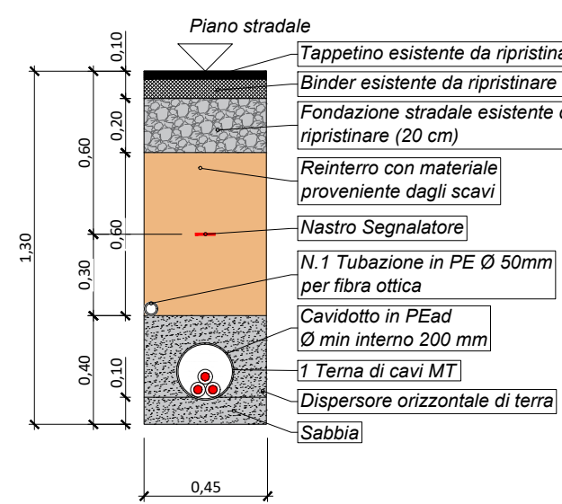
SEZIONE DI POSA "1AN" STRADA ASFALTATA ESISTENTE
