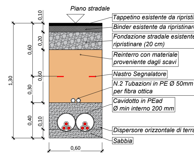
SEZIONE DI POSA "2AN" STRADA ASFALTATA ESISTENTE
