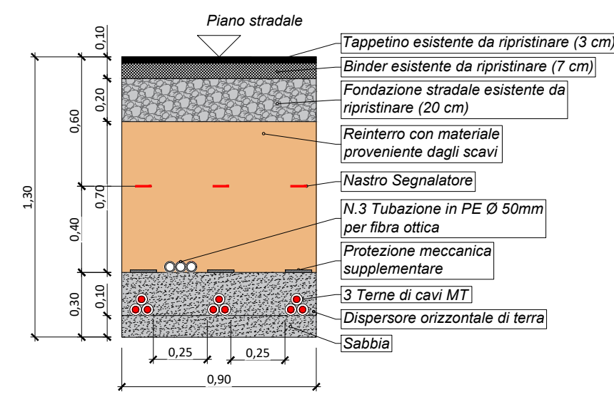
SEZIONE DI POSA "3AN" STRADA ASFALTATA ESISTENTE
