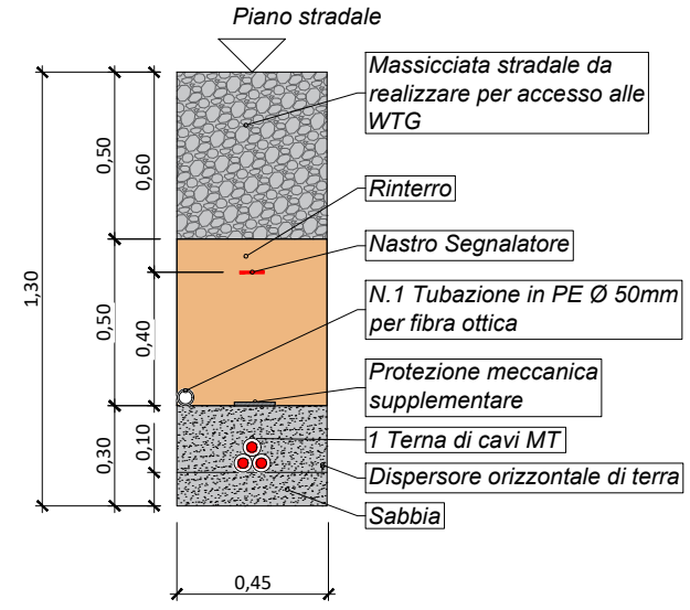
SEZIONE DI POSA "1AM" STRADA ASFALTATA ESISTENTE
