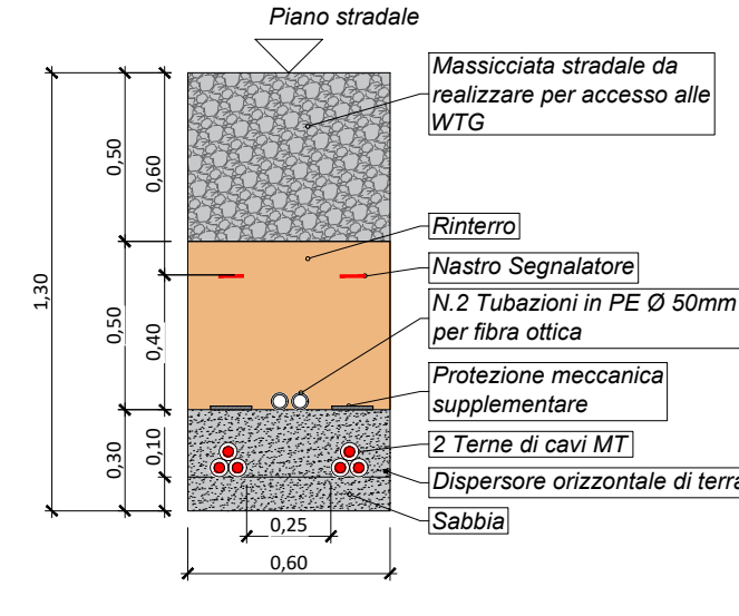
SEZIONE DI POSA "2AM" STRADA ASFALTATA ESISTENTE
