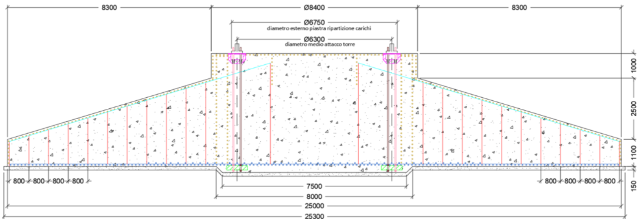
Figura 1 – Sezione plinto di fondazione.
