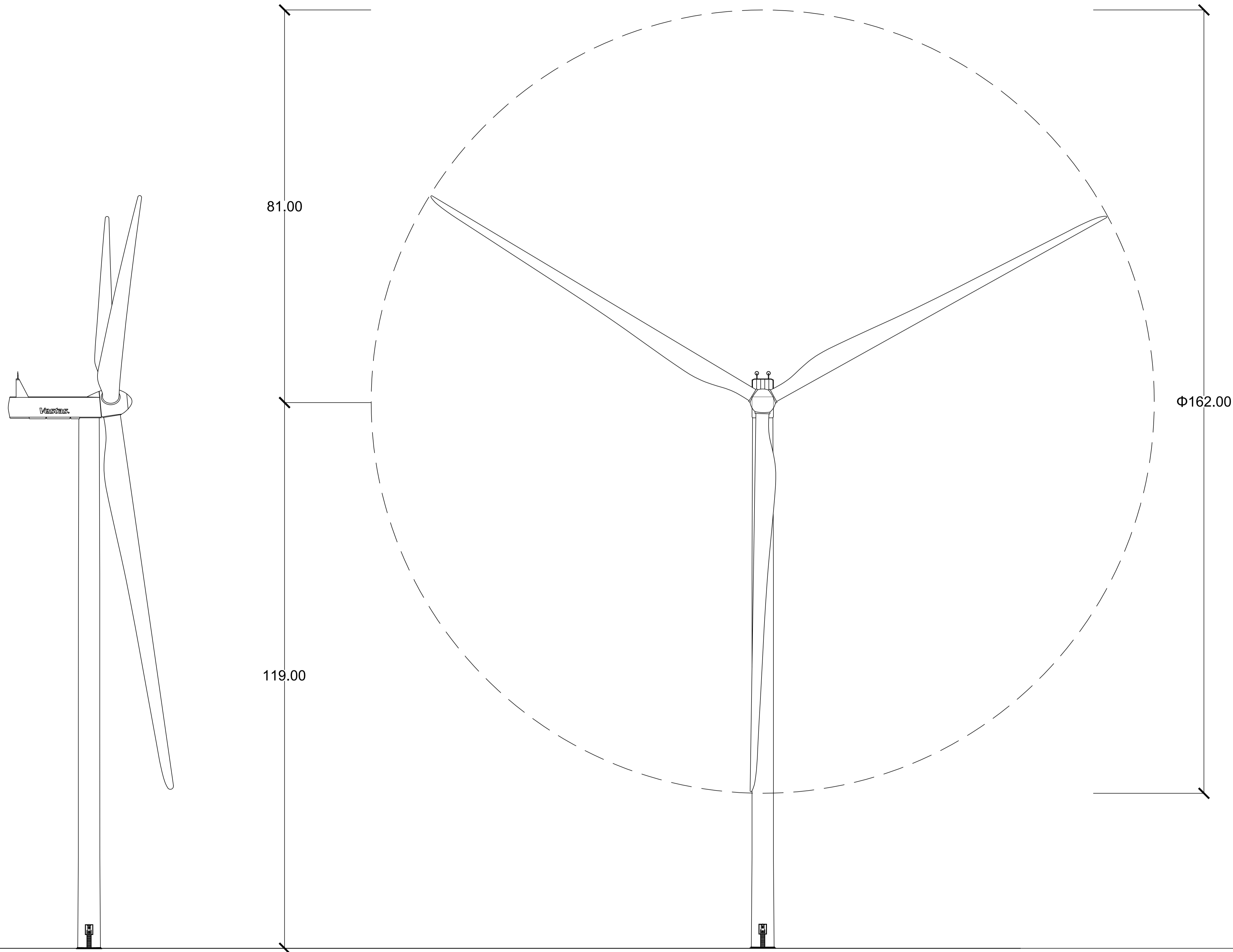
VISTA FRONTALE - SCALA 1:400
