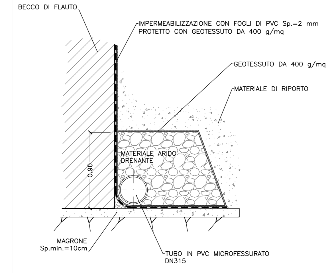
PARTICOLARE "A" SCALA 1:25
