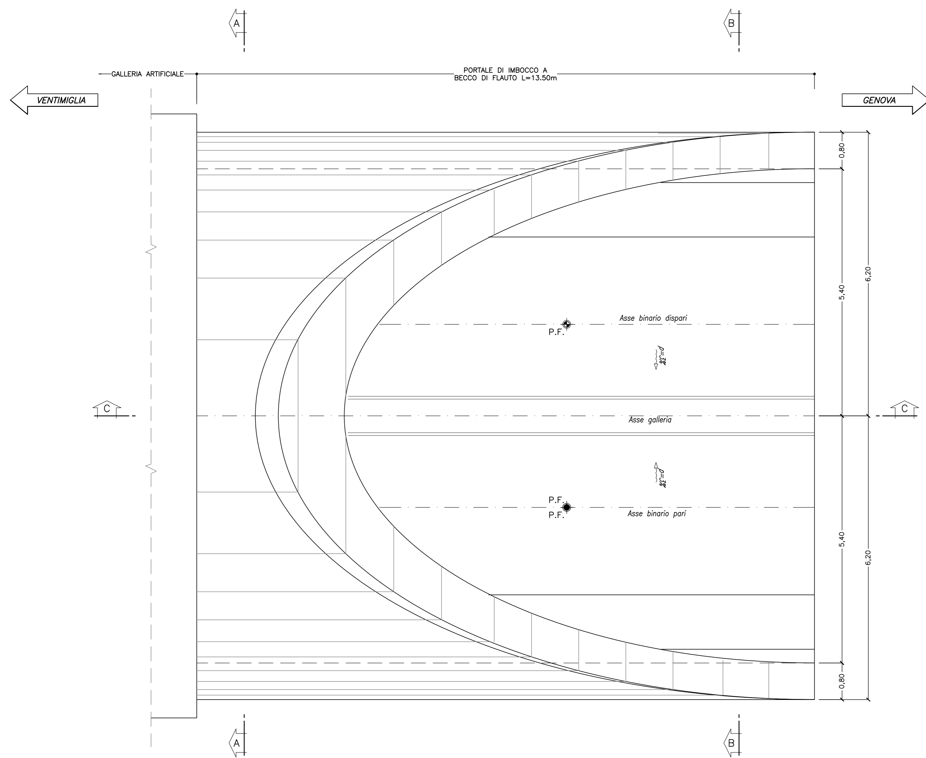
PIANTA SCALA 1:50
