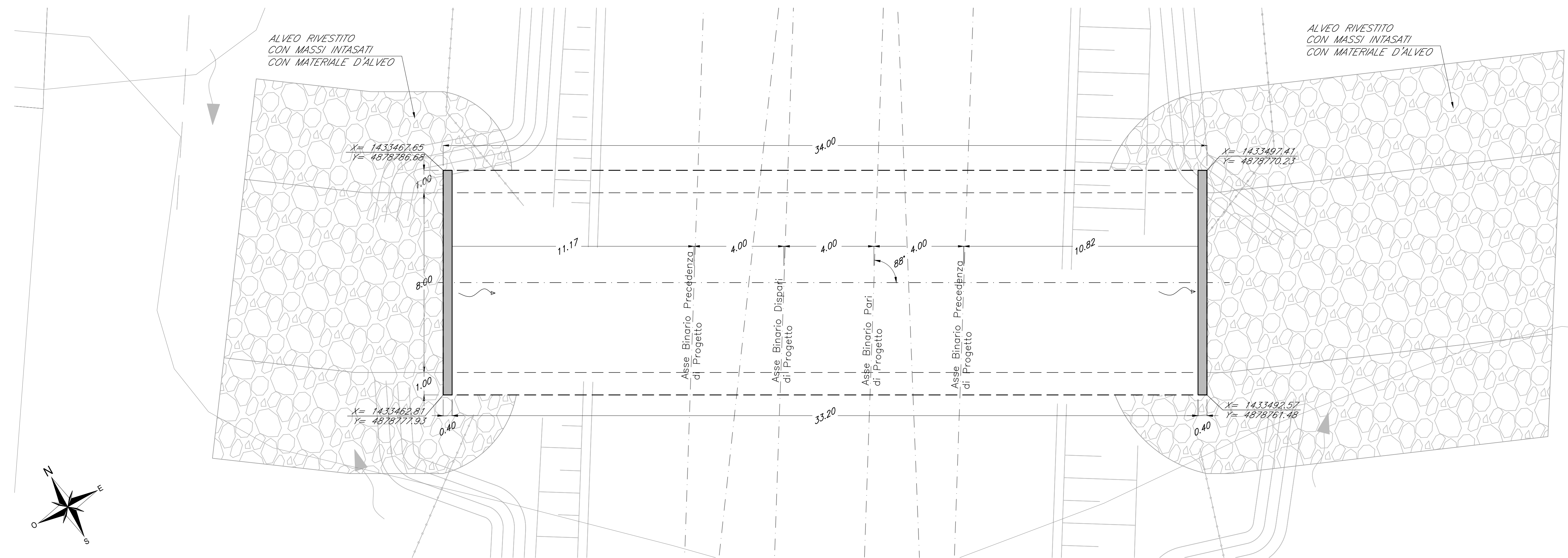
TOMBINO SCATOLARE RIO DELLA VALLETTA - PLANIMETRIA Scala: 1:100
