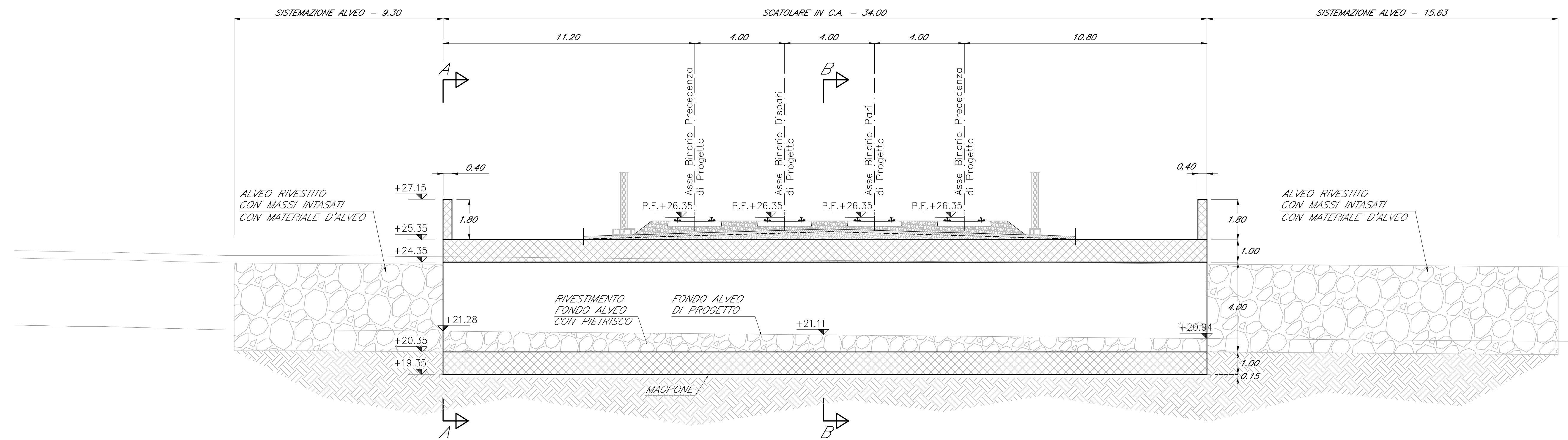
TOMBINO SCATOLARE RIO DELLA VALLETTA - PROFILO LONGITUDINALE Scala: 1:100
