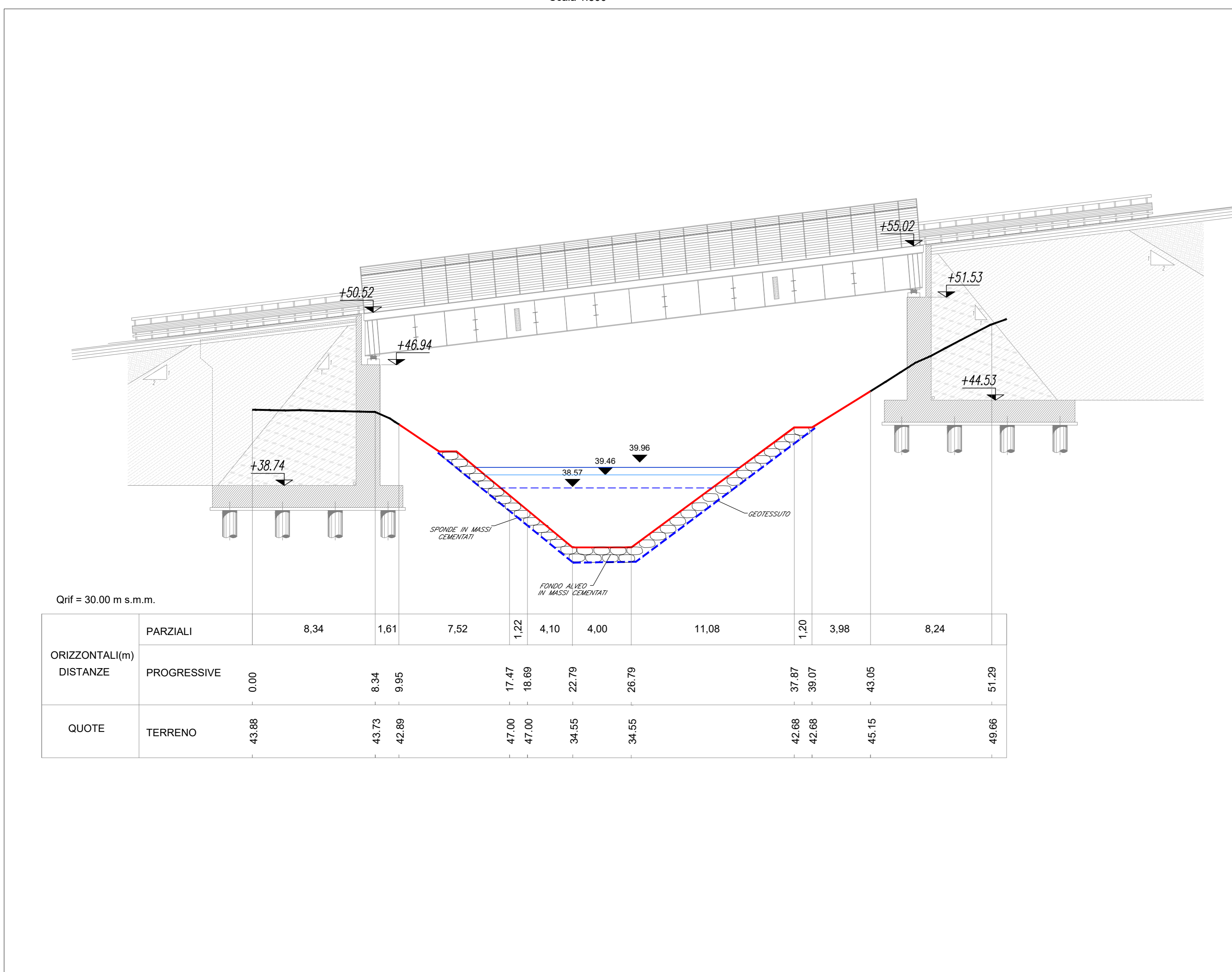
SEZIONI ALVEO RIO AVEGLIA IN CORRISPONDENZA DELLA NUOVA VIABILITA' NVX3
