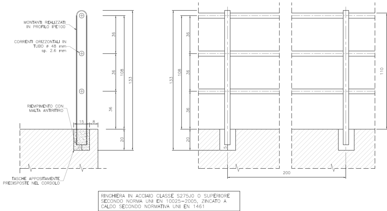
Figura 6: Parapetto metallico
