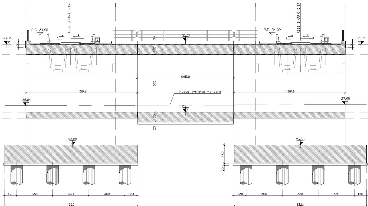
Figura 3: Scatolare - Sezione longitudinale
