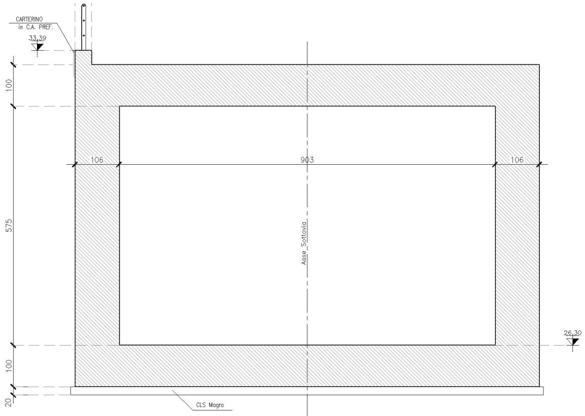
Figura 4: Scatolare - Sezione trasversale
