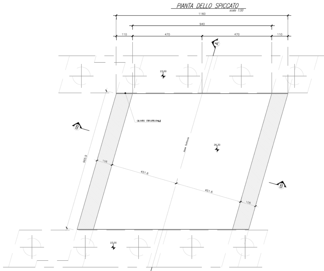
Figura 5: Scatolare - Pianta superiore
