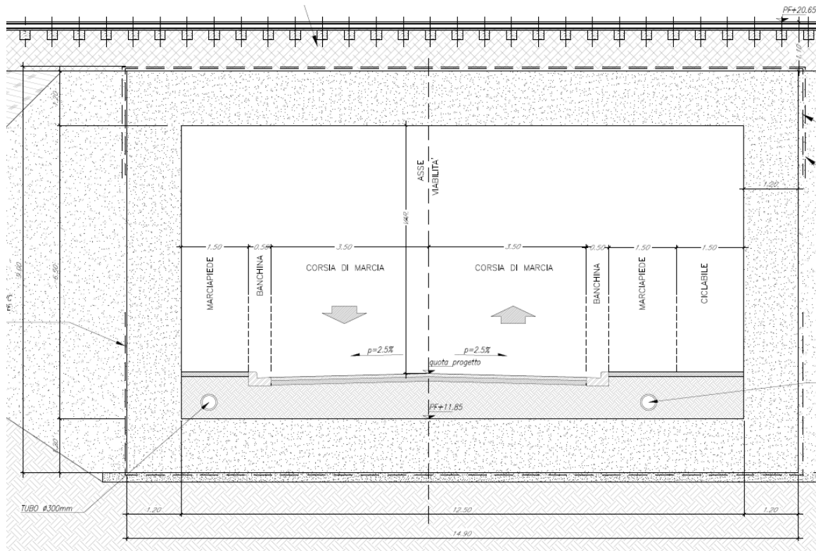
Figura 4: Scatolare - Sezione trasversale
