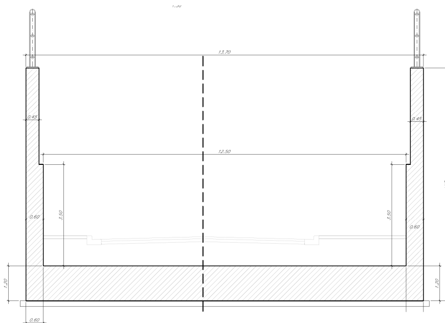
Figura 7: Muro di sbocco/imbocco - Sezione trasversale
