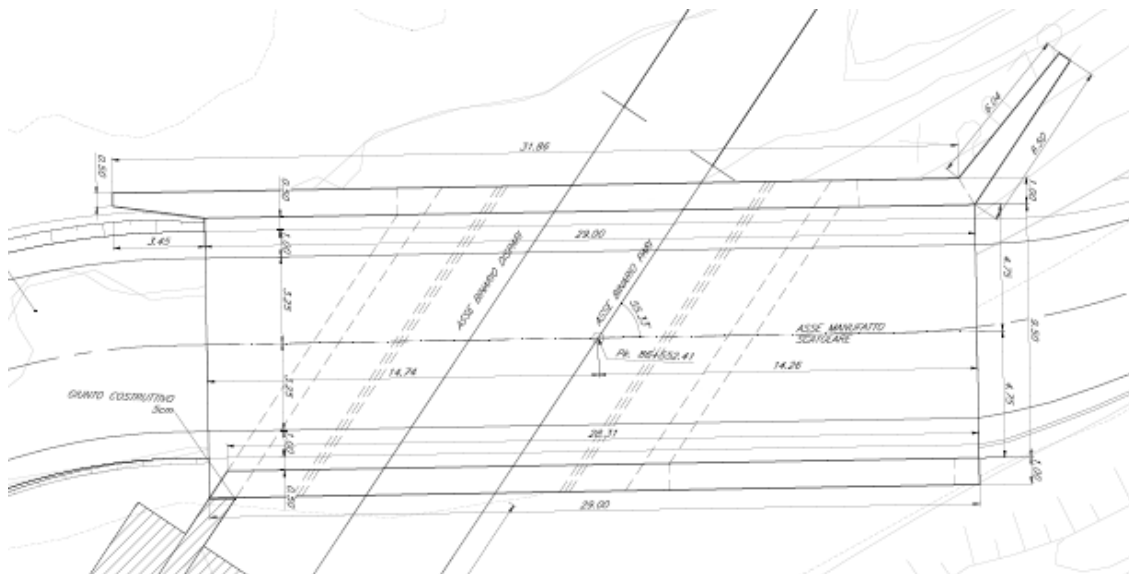
Figura 5: Scatolare - Pianta superiore
