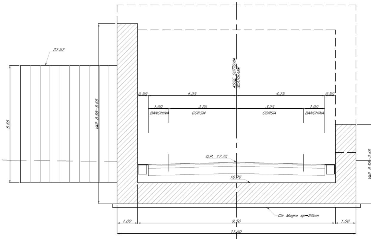
Figura 7: Muro di sbocco/imbocco - Sezione trasversale
