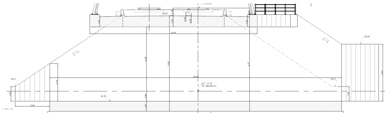
Figura 3: Scatolare - Sezione longitudinale
