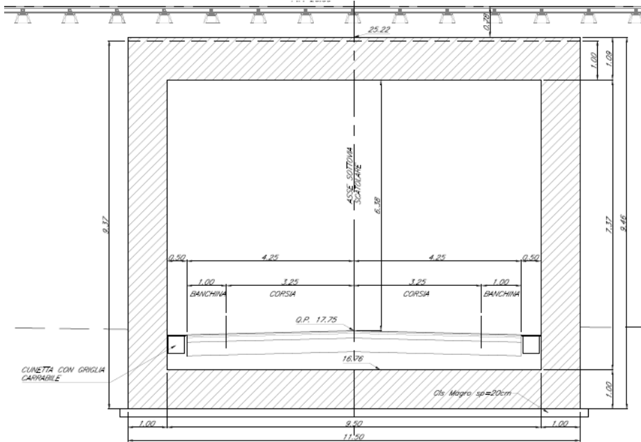
Figura 4: Scatolare - Sezione trasversale
