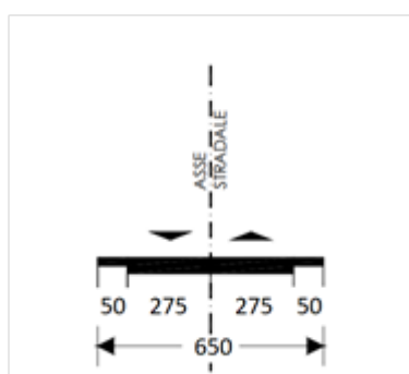
Figura 4 - Sezione tipo
