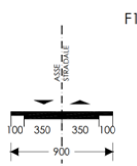
Figura 5 – Sezione tipo di progetto
