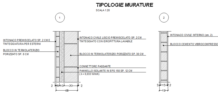
Figura 5: dettagli murature di tamponamento e pareti interne
