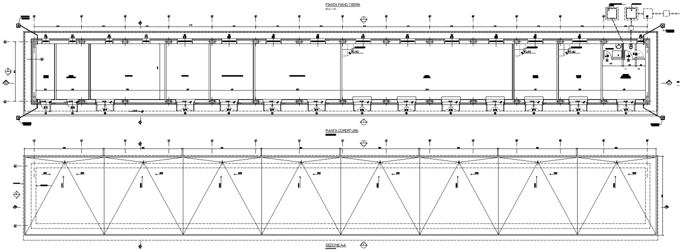
Figura 3 pianta piano terra e copertura
