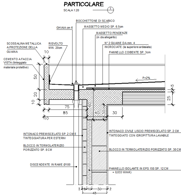
Figura 7: dettaglio gronda
