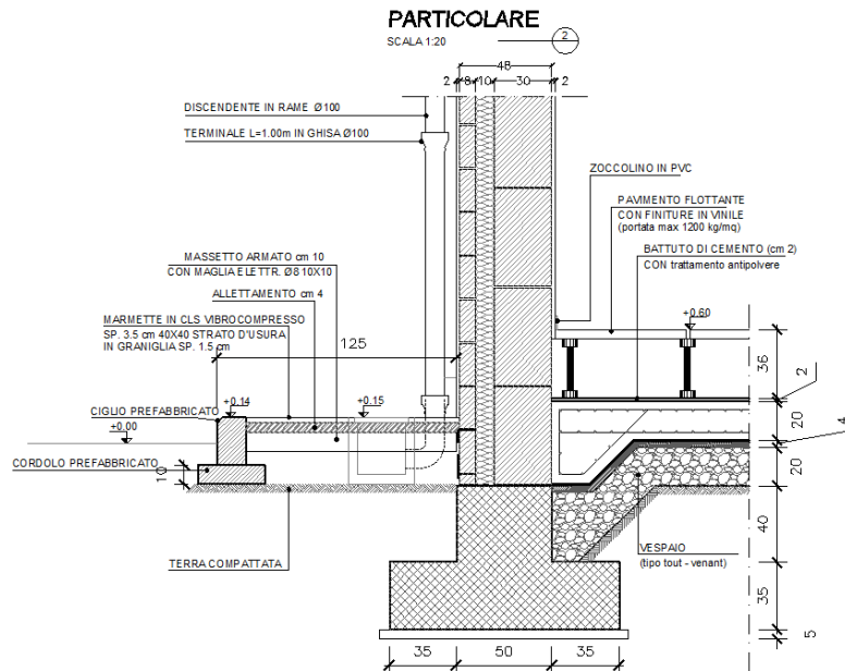
Figura 6: dettaglio nodo di fondazione
