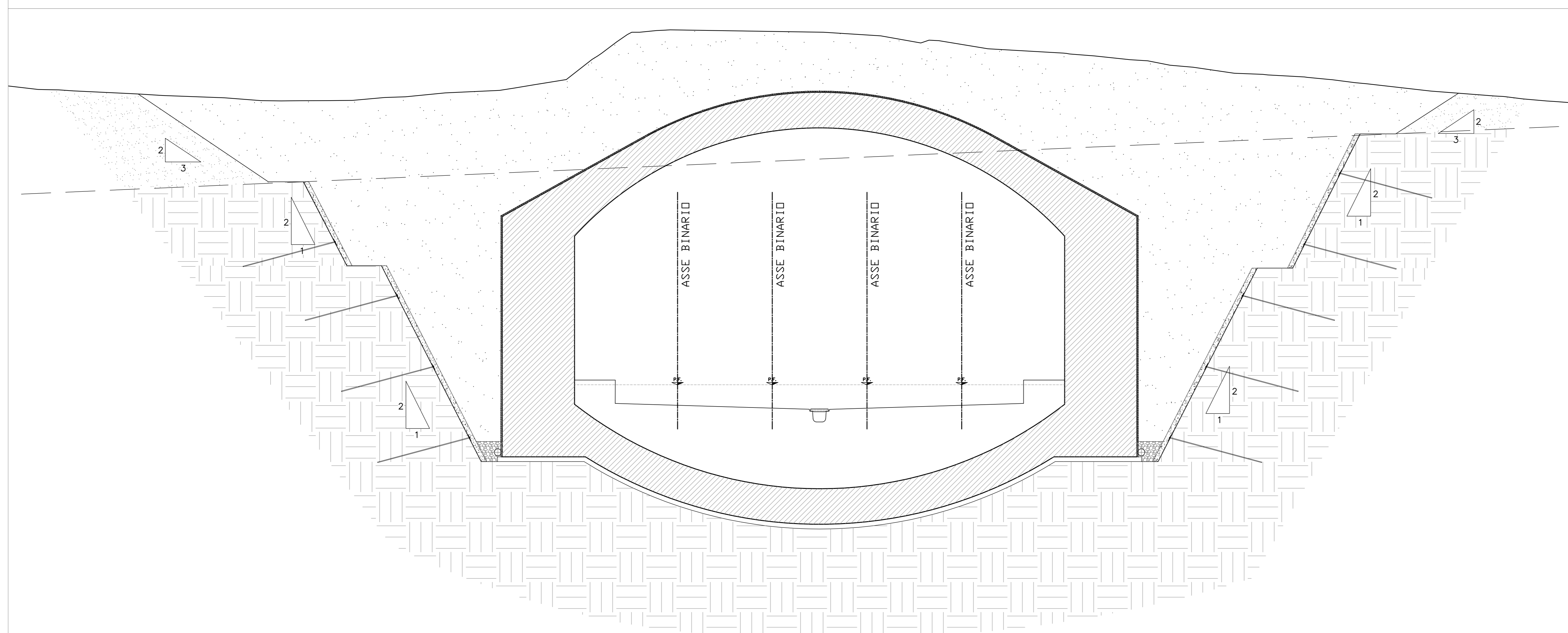
FASE "3" Realizzazione opere di finitura e ripristino del profilo terreno preesistente
