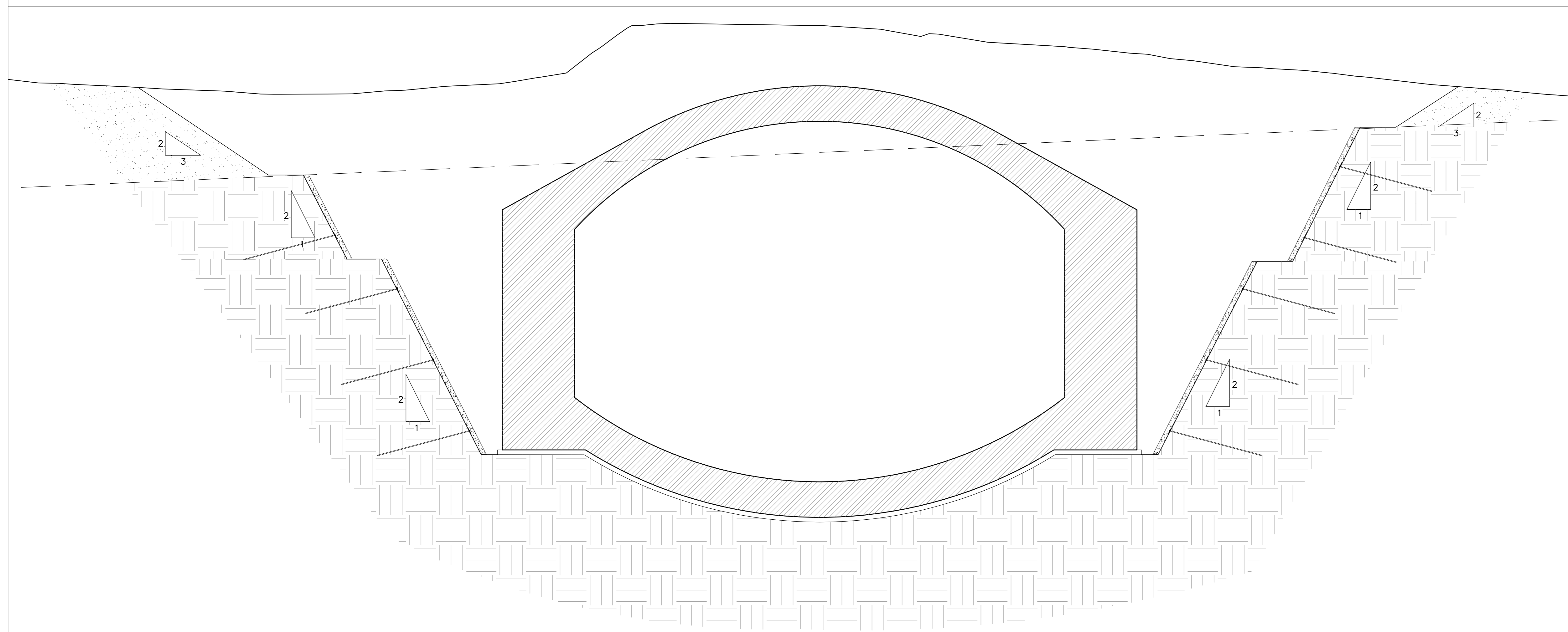
FASE "2" Realizzazione galleria sezione policentrica.
