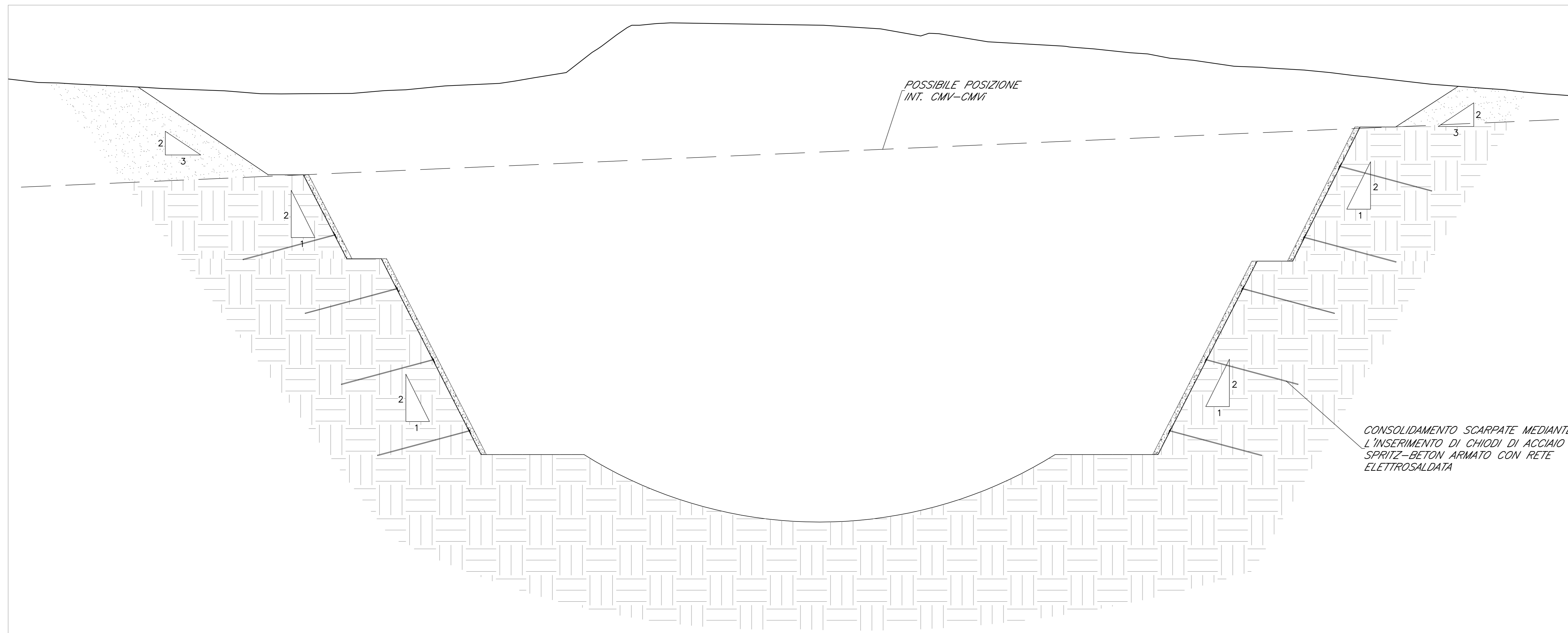
FASE "1" Scavo fino a quota fondo galleria.
