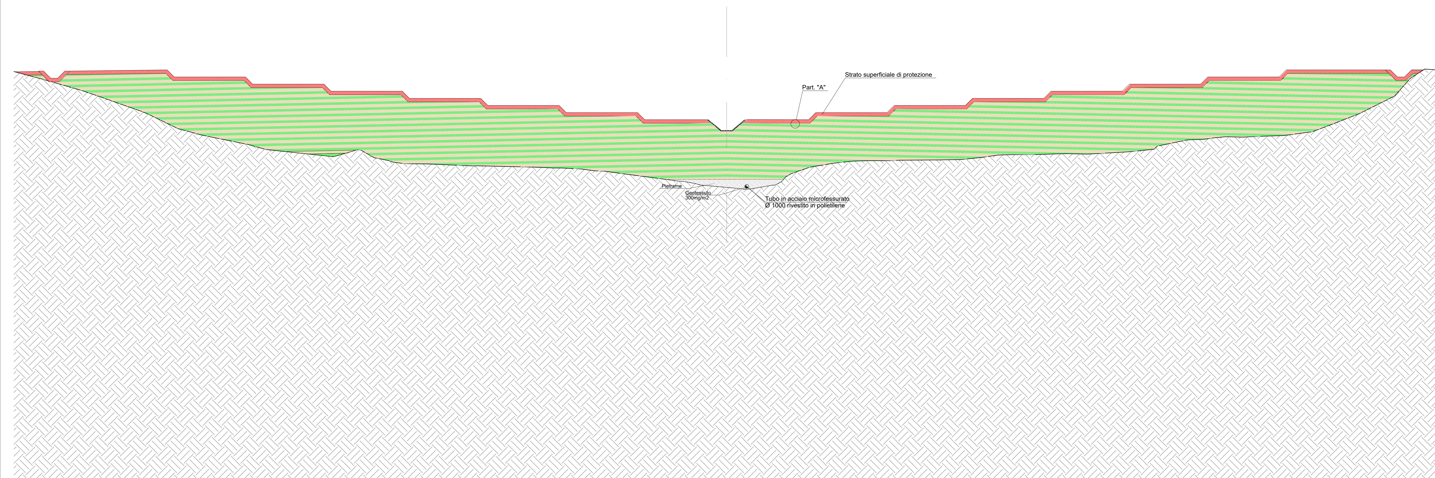
Particolare "A": STRATI RILEVATO
