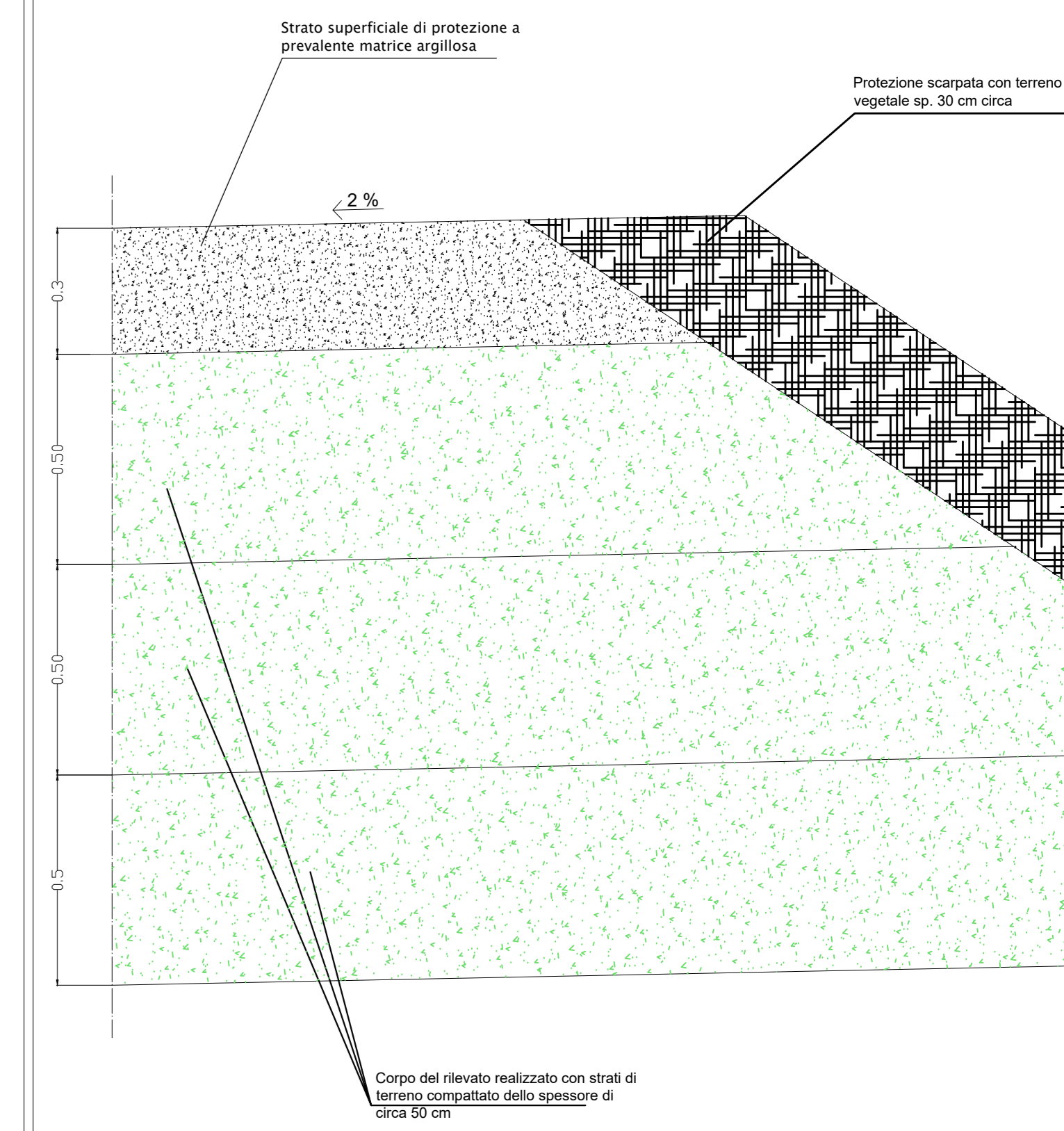
Particolare "A": STRATI RILEVATO
