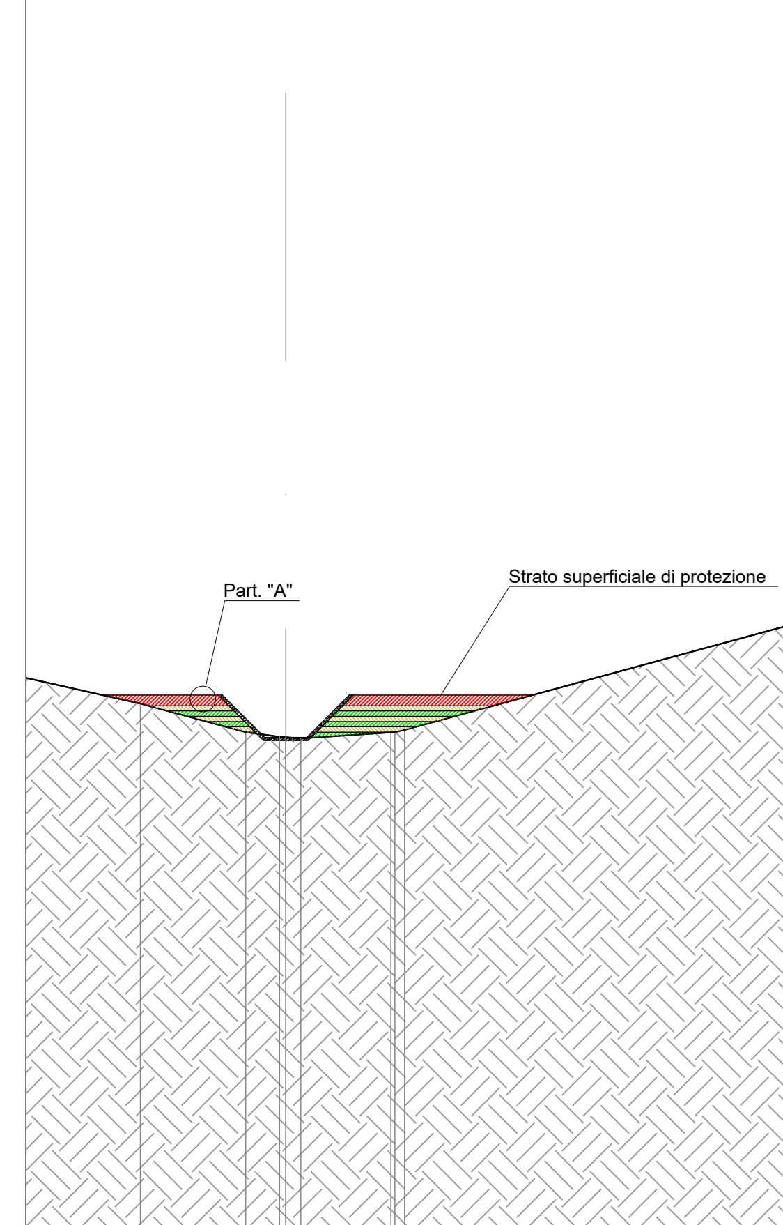
SEZIONE TIPO 1
