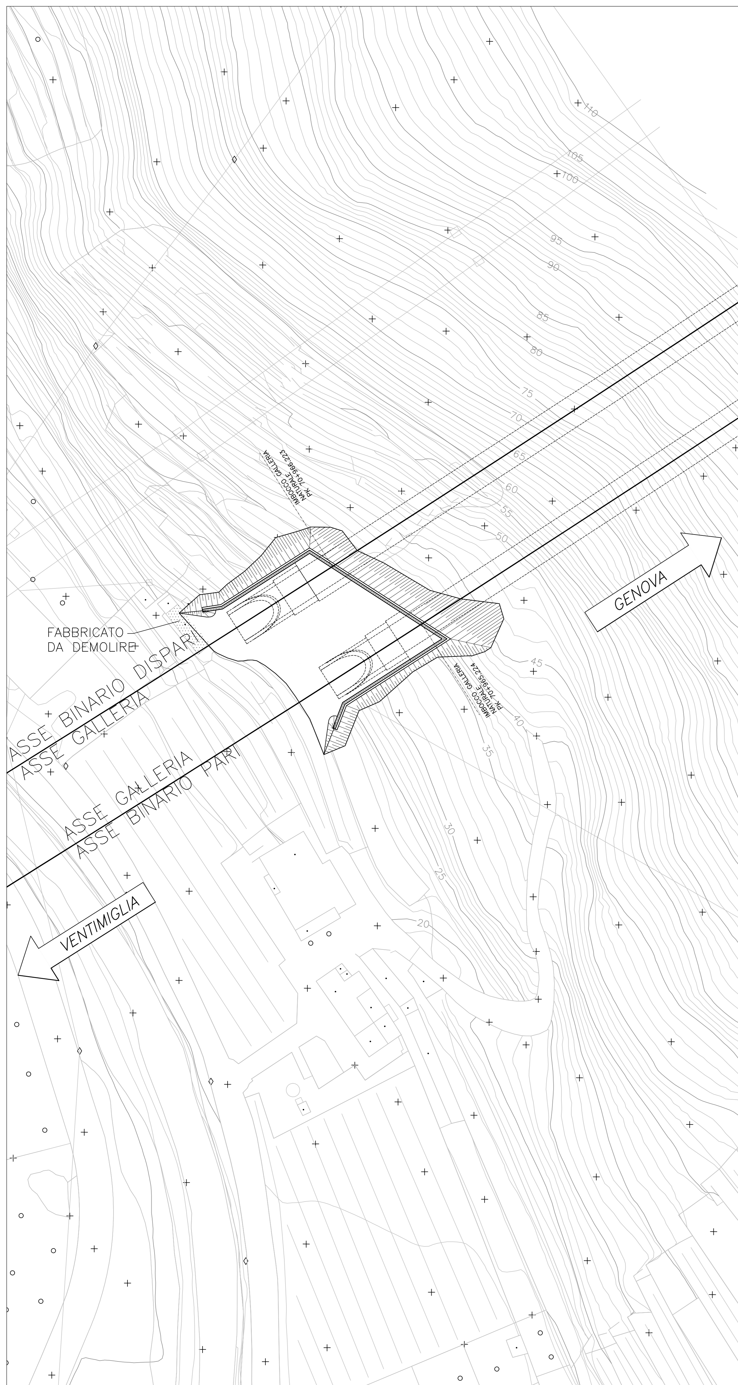
PLANIMETRIA GENERALE SCALA 1:500
