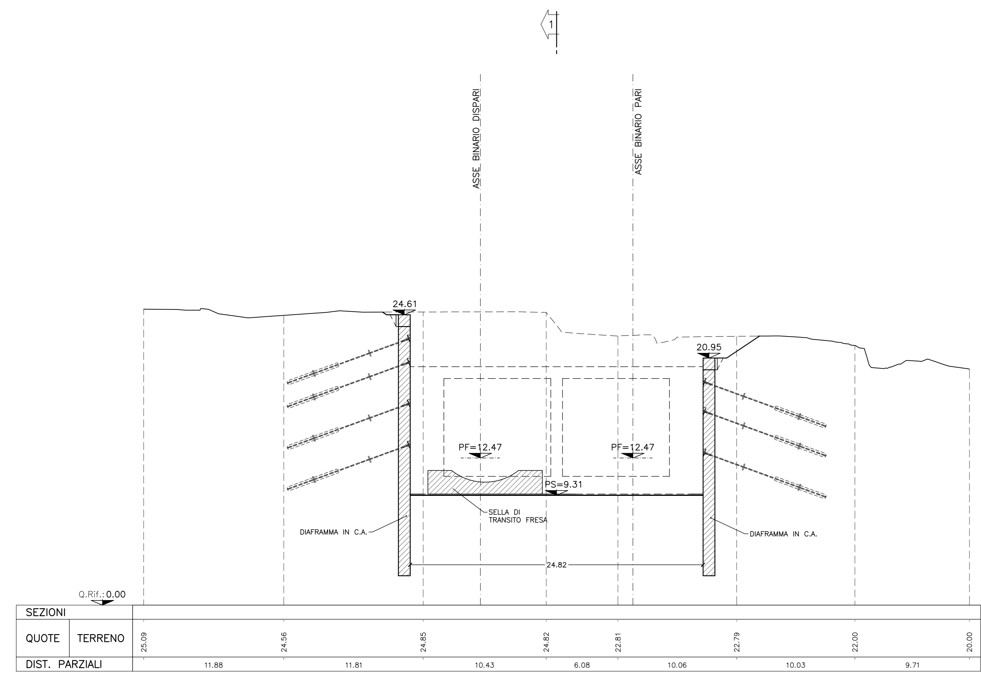
SEZIONE 3-3 SCALA 1:200 INIZIO DIMA
