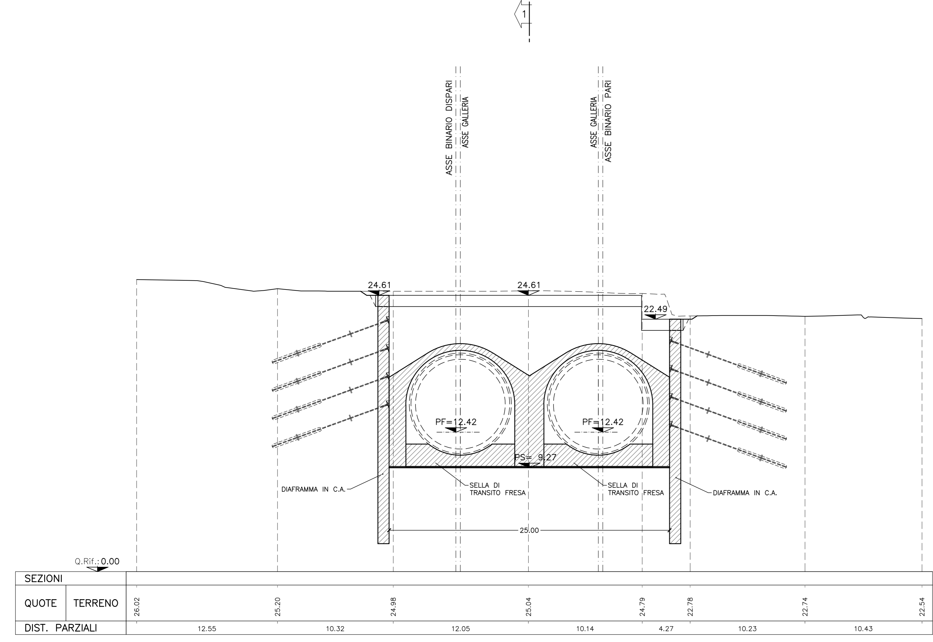
SEZIONE 2-2 SCALA 1:200 IMBOCCO GALLERIA NATURALE
