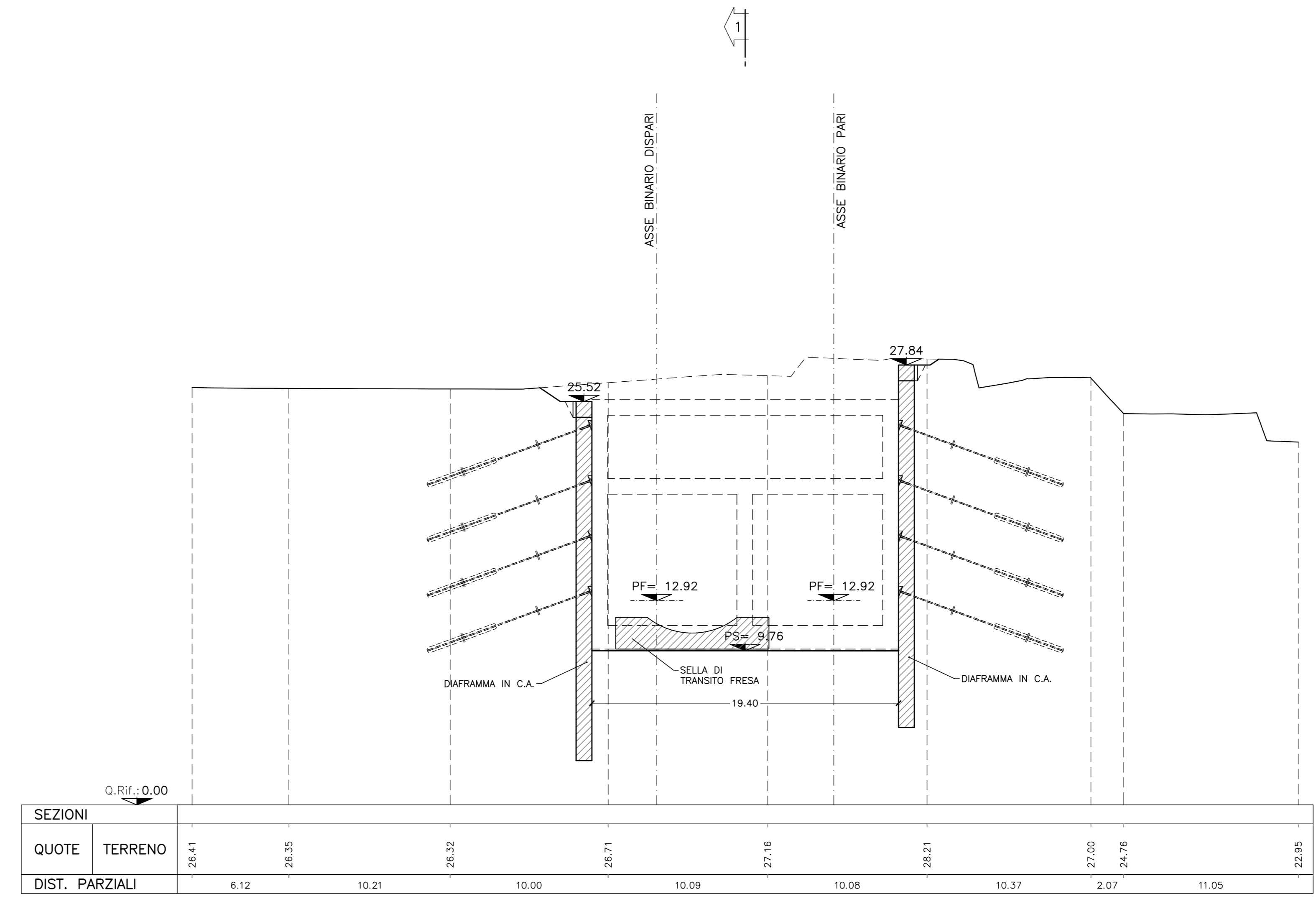
SEZIONE 4-4 SCALA 1:200 GALLERIA ARTIFICIALE
