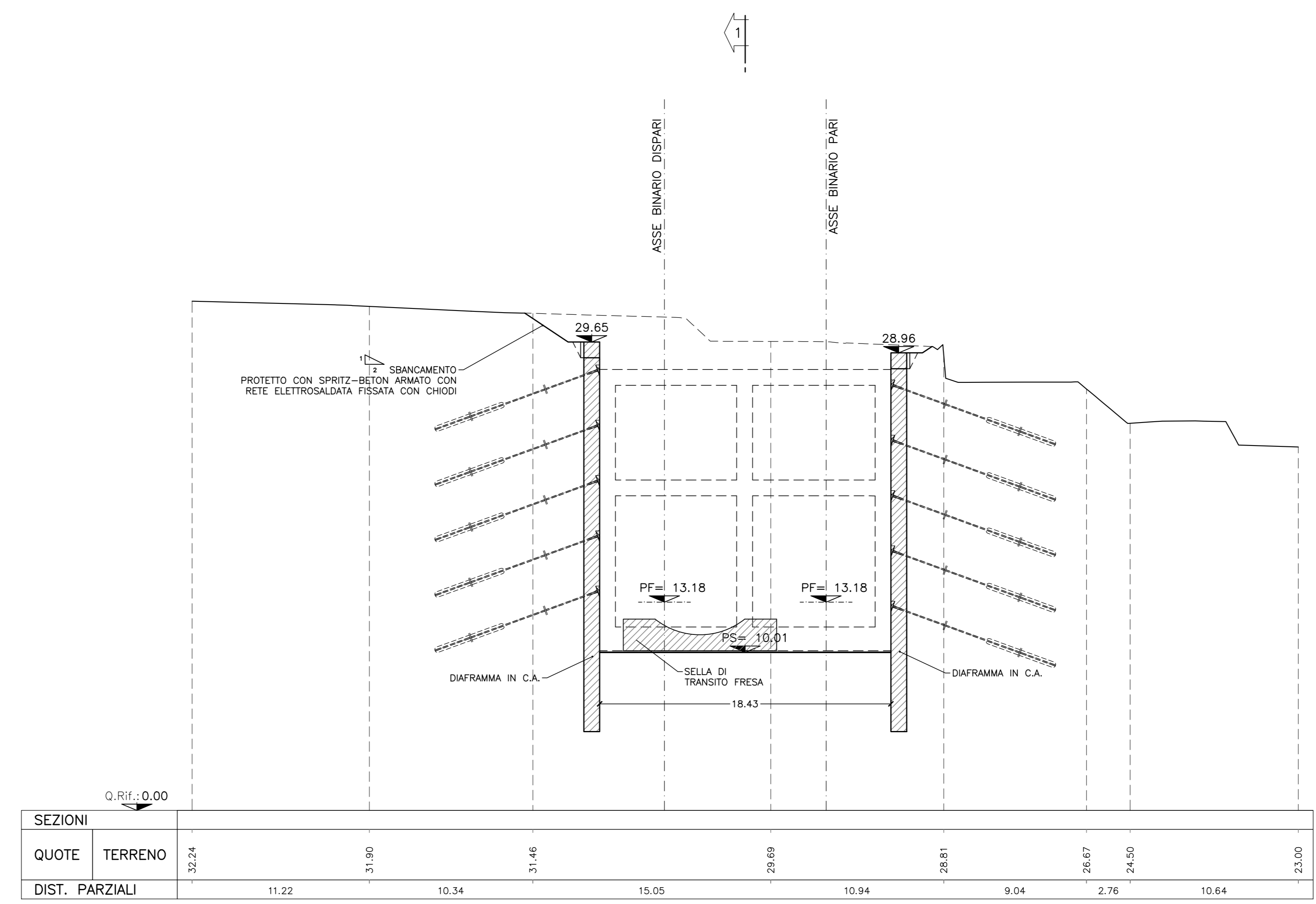
SEZIONE 5-5 SCALA 1:200 GALLERIA ARTIFICIALE
