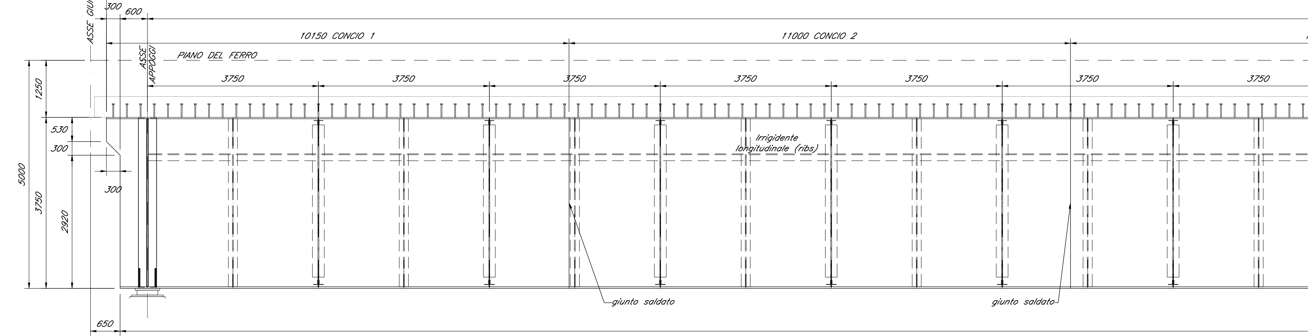
1/2 PROSPETTO LONGITUDINALE Scala 1:50
