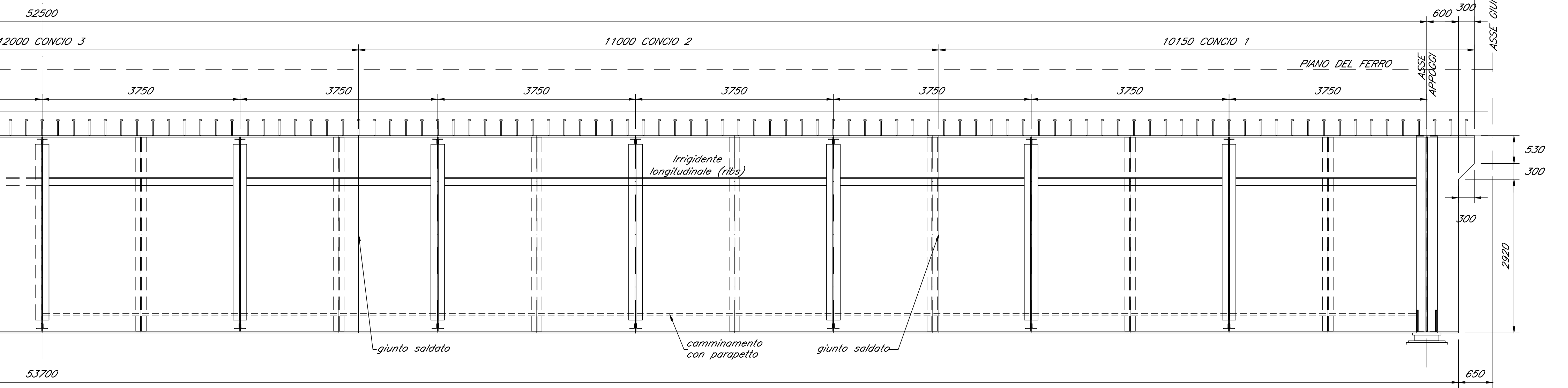
1/2 SEZIONE LONGITUDINALE Scala 1:50
