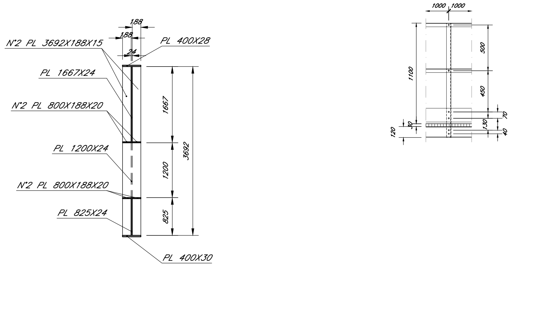
DETTAGLIO CAMMINAMENTO CON PARAPETTO Scala 1:25
