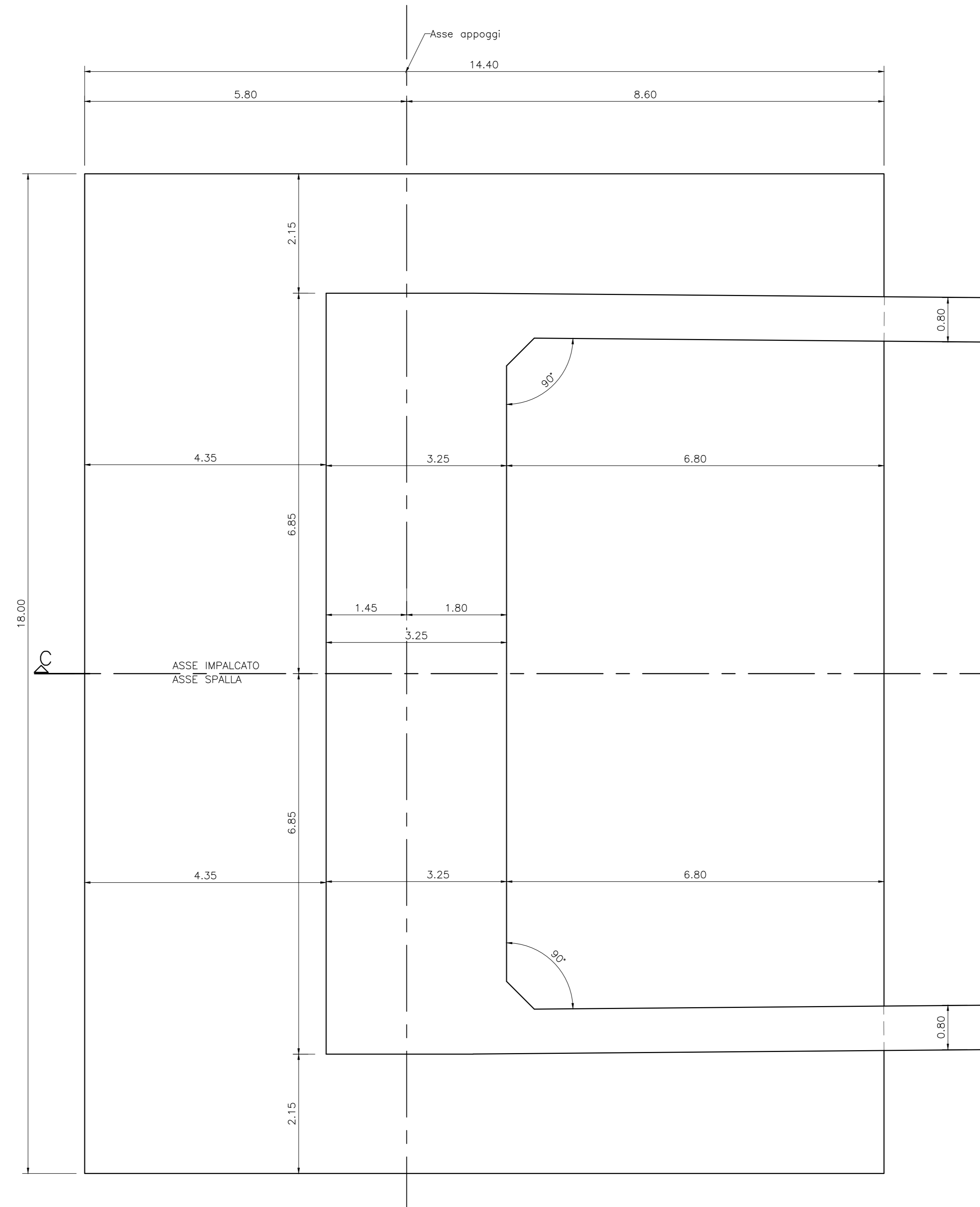
PIANTA "E" SCALA 1:50
