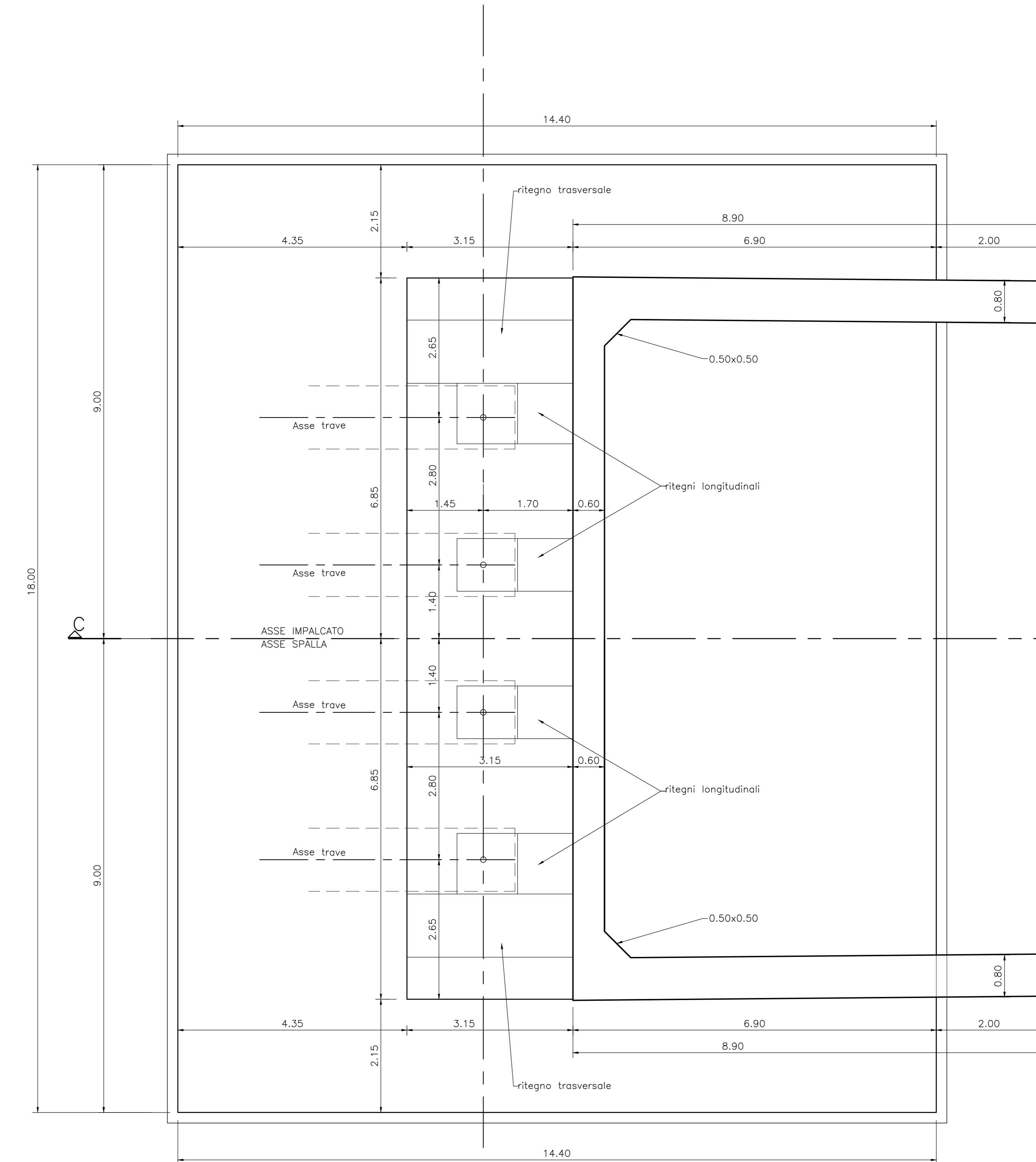
PIANTA "B" SCALA 1:50
