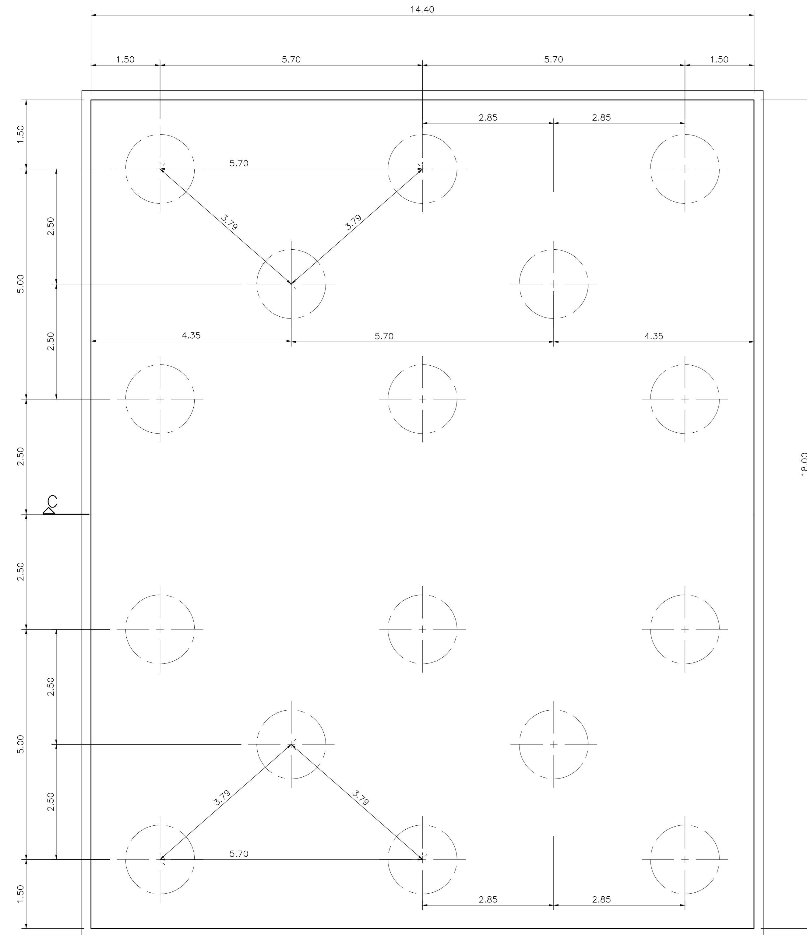
PIANTA "A" SCALA 1:50
