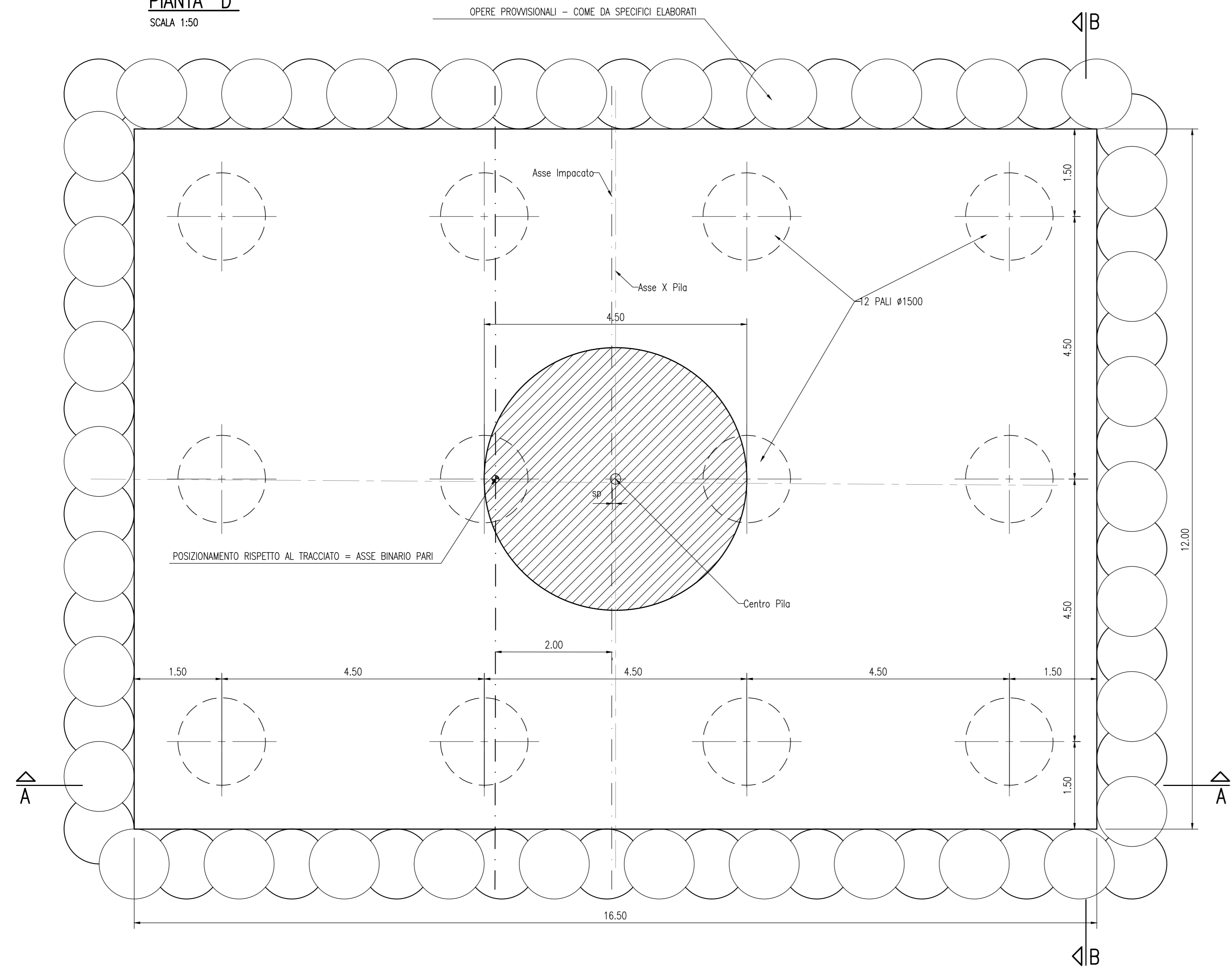
PIANTA "D" SCALA 1:50
