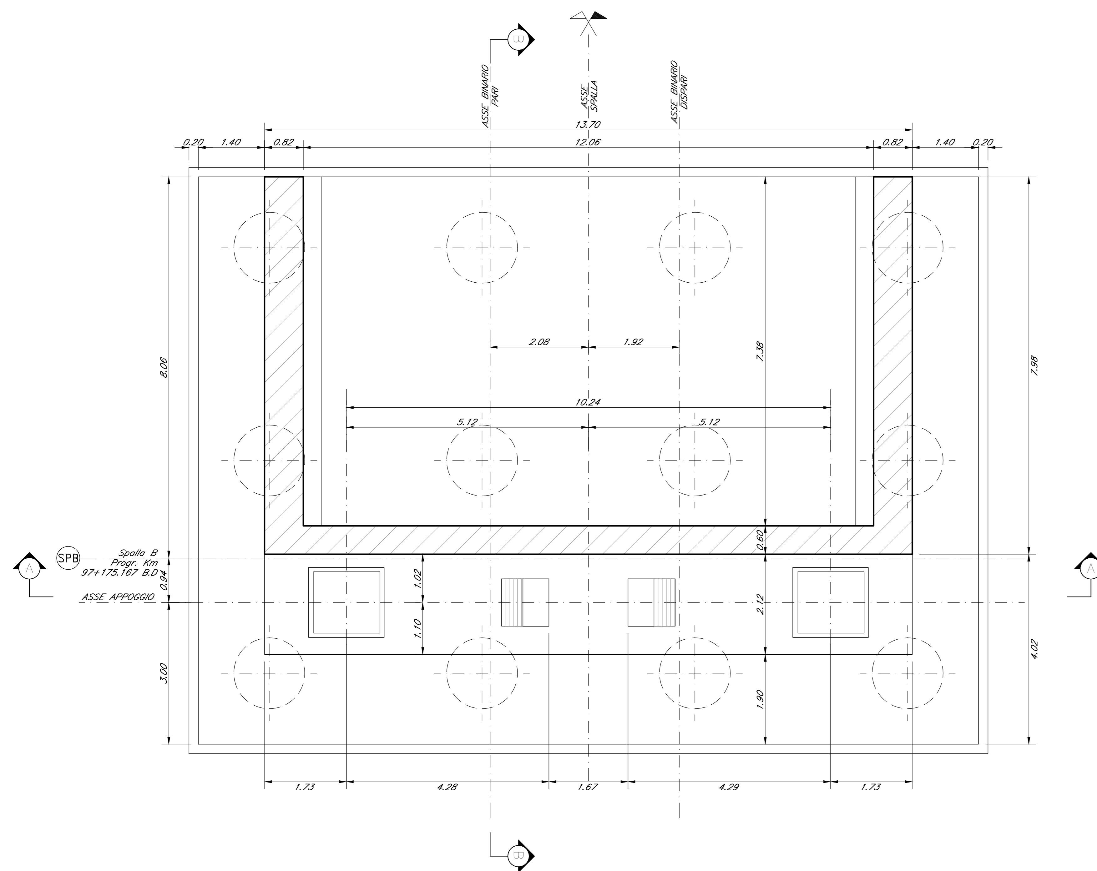
PIANTA - SEZIONE 3-3 Scala 1:50
