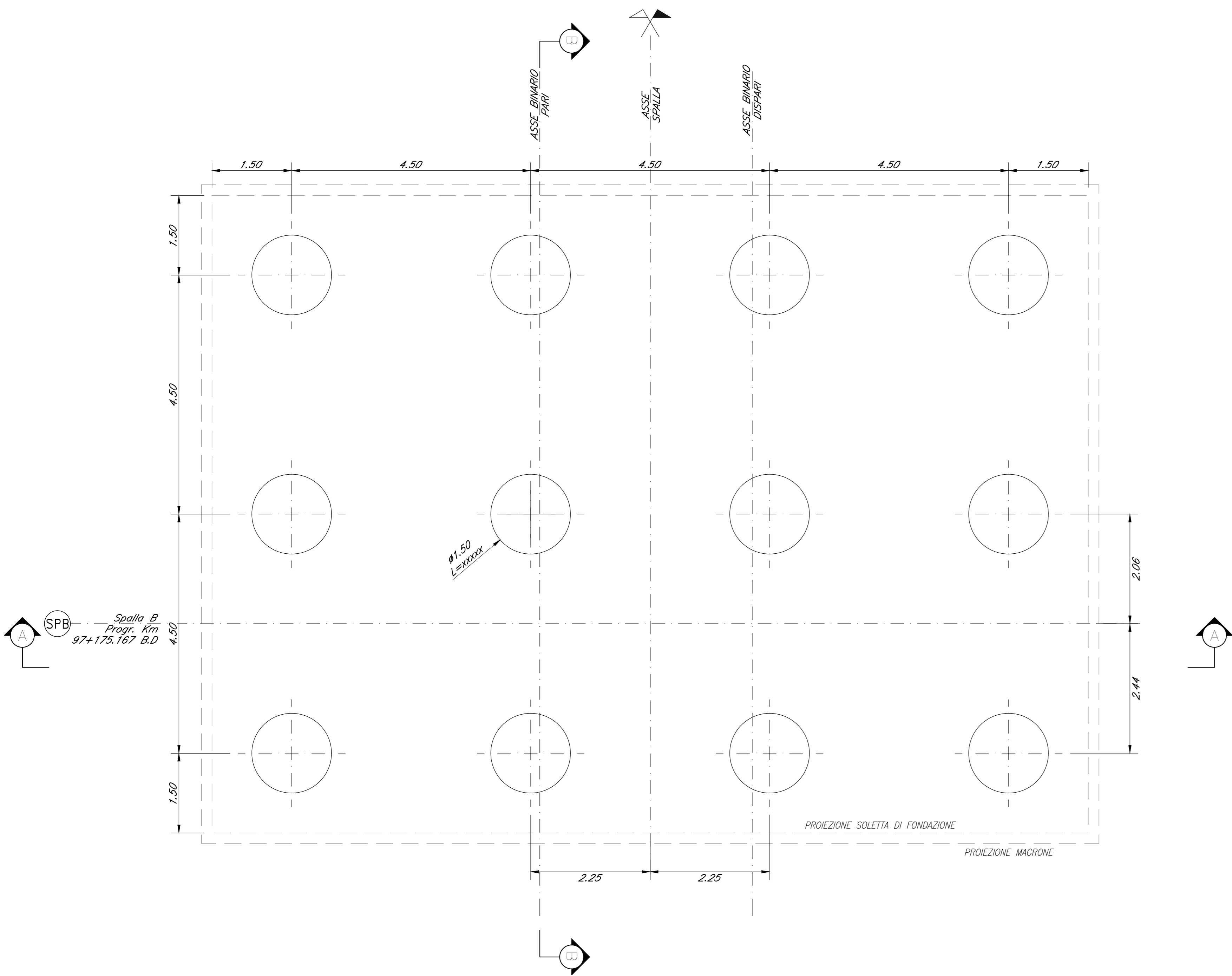
SEZIONE 1-1 PIANTA PALI Scala 1:50
