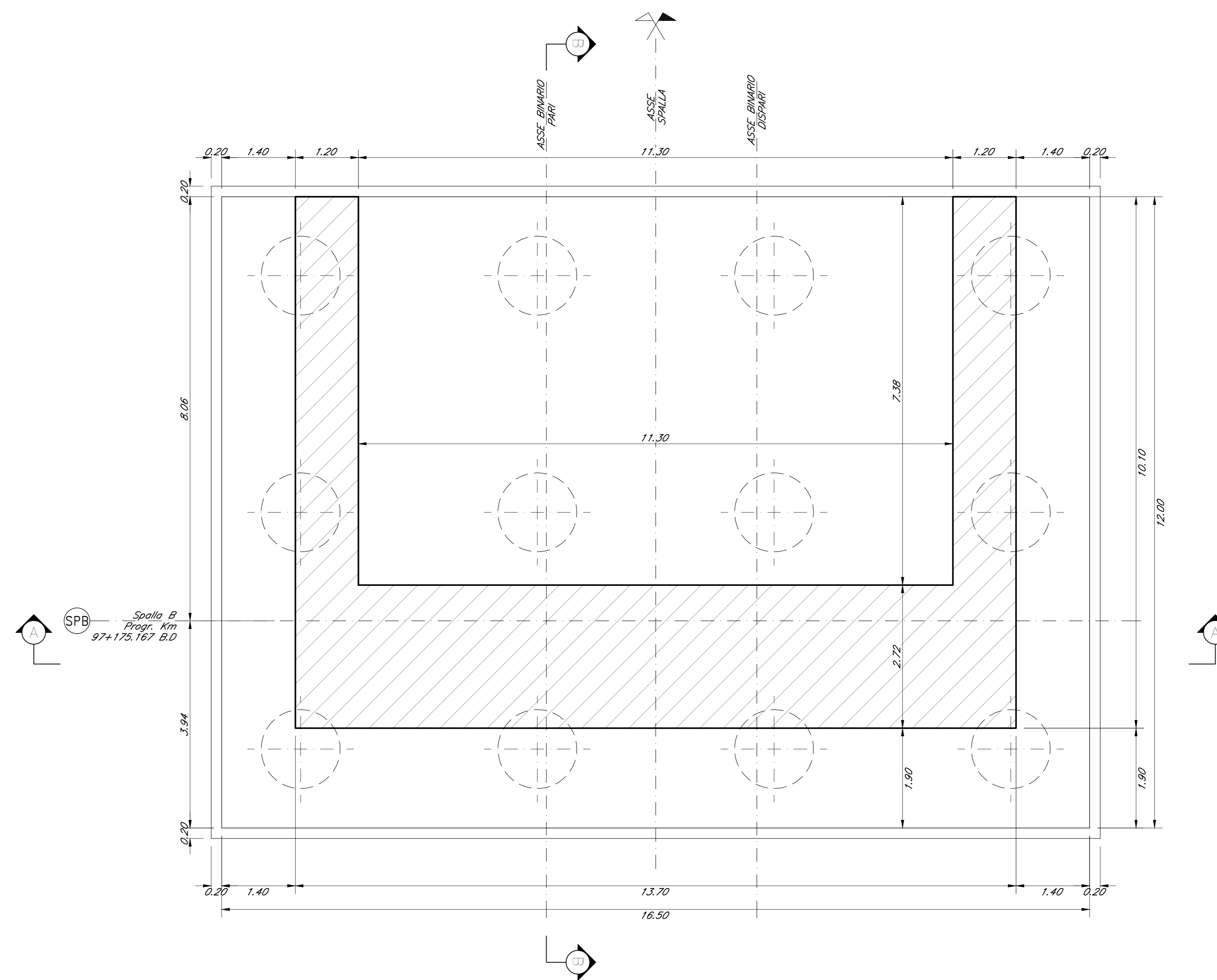
PIANTA - SEZIONE 2-2 Scala 1:50
