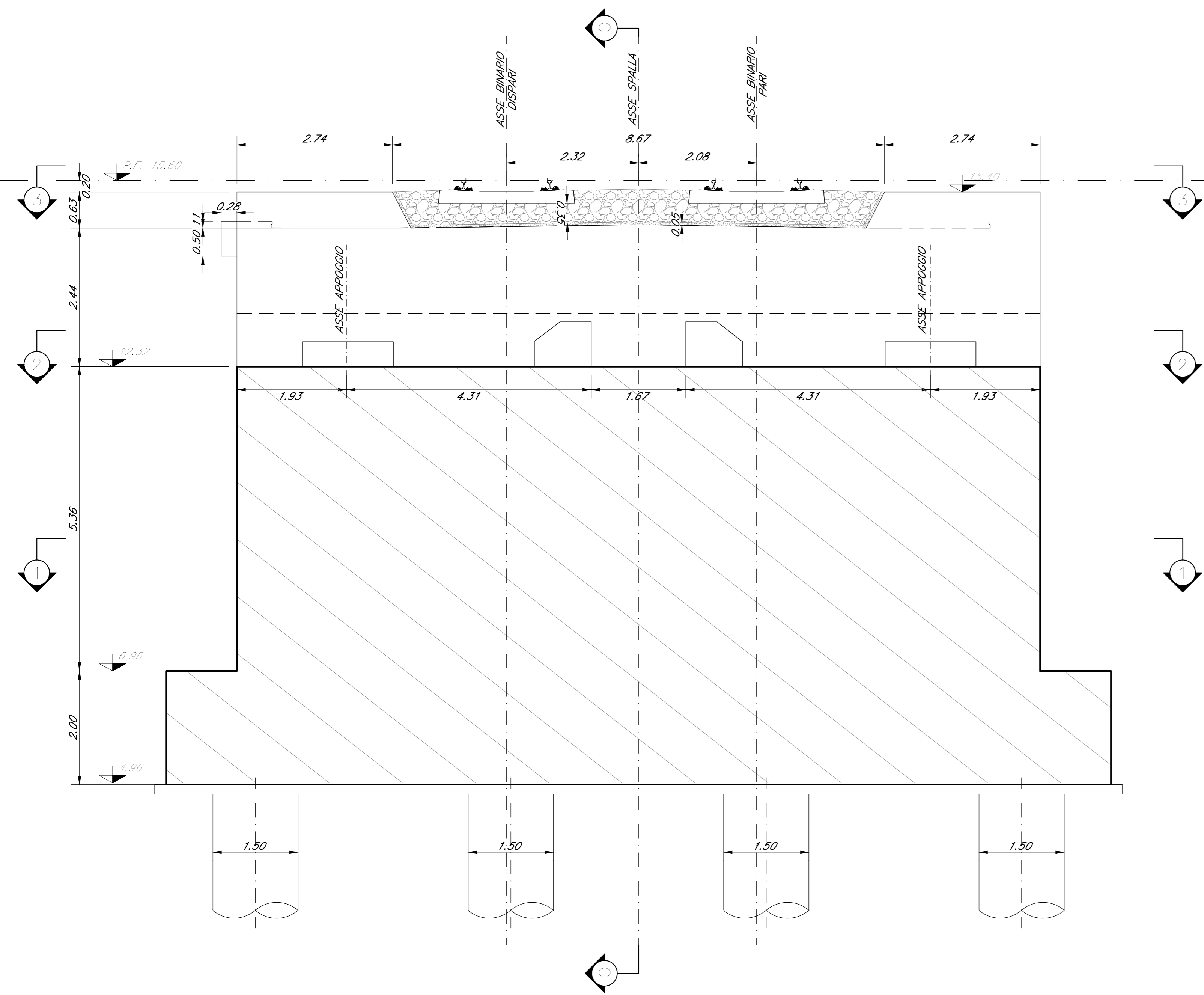
SEZIONE TRASVERSALE A-A Scala 1:50
