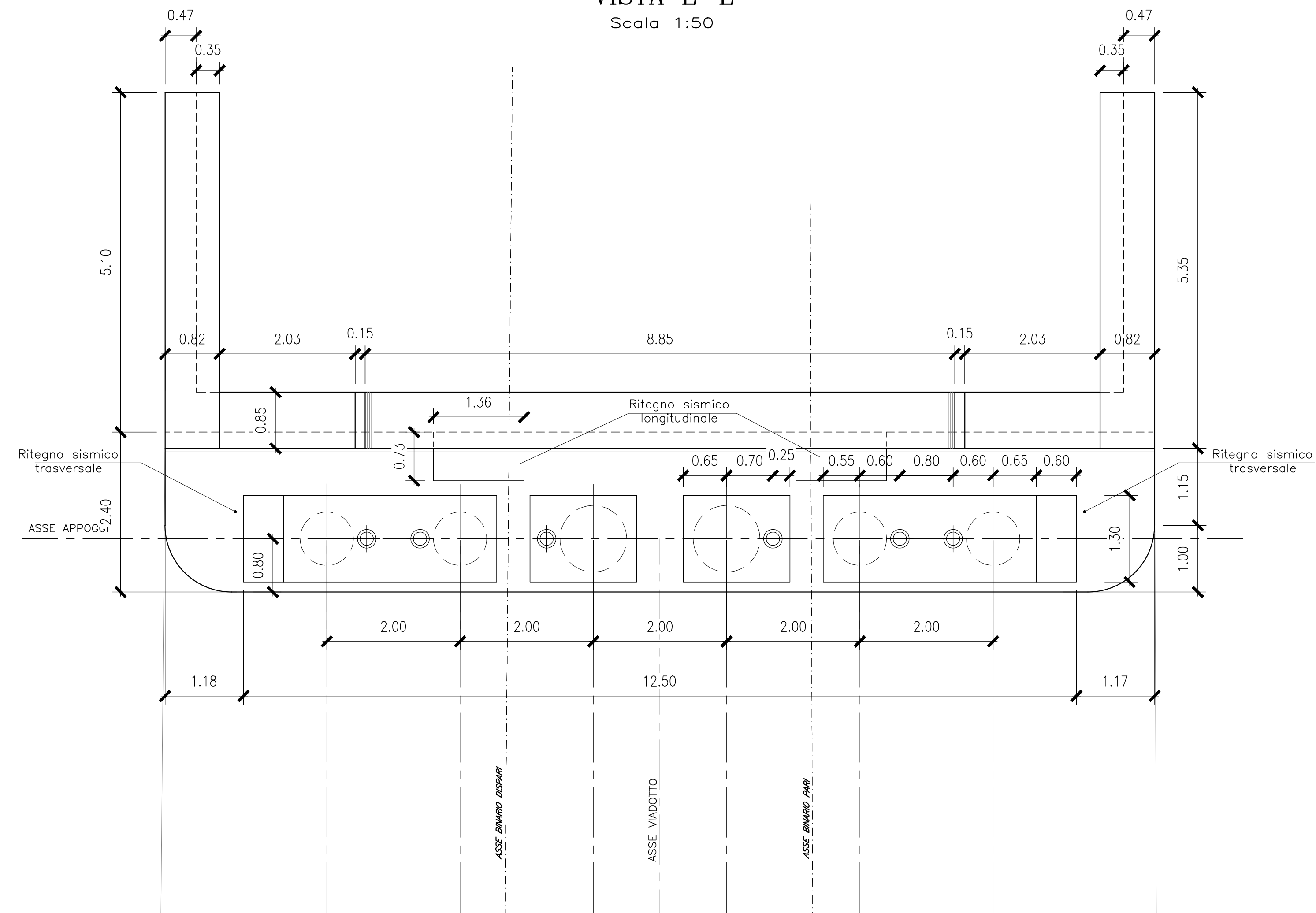
VISTA E-E Scala 1:50
