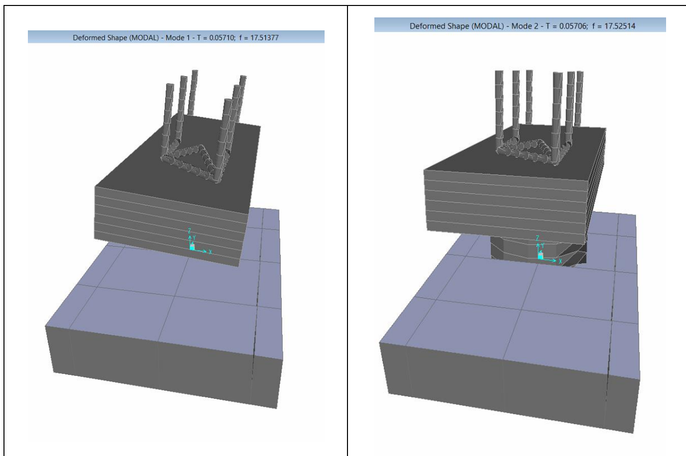
Figura 3: Modello FEM – Analisi Modale (50% rigidezza)
