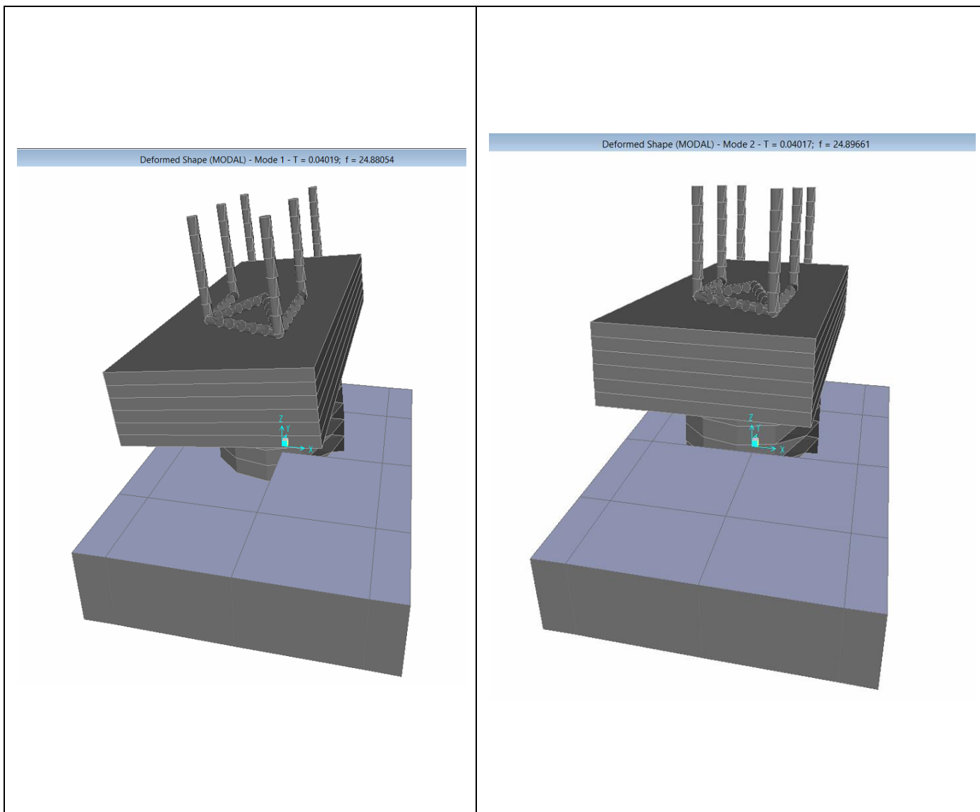
Figura 2: Modello FEM – Analisi Modale (100% rigidezza)
