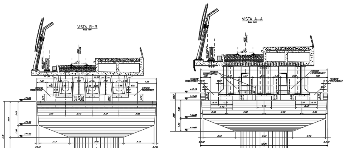
Figura 2 - sezione trasversale impalcato sx e dx
