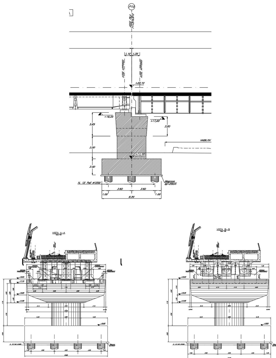
Figura 5 – prospetti pila
