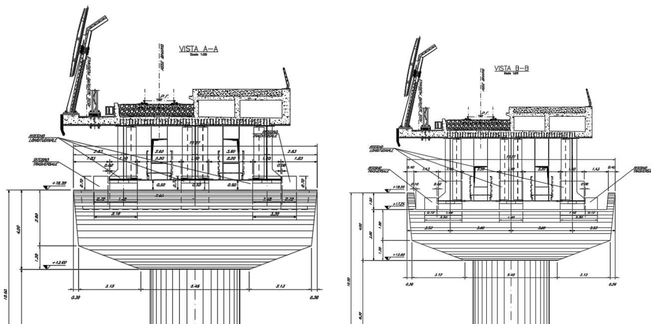
Figura 2 - sezione trasversale impalcato sx e dx
