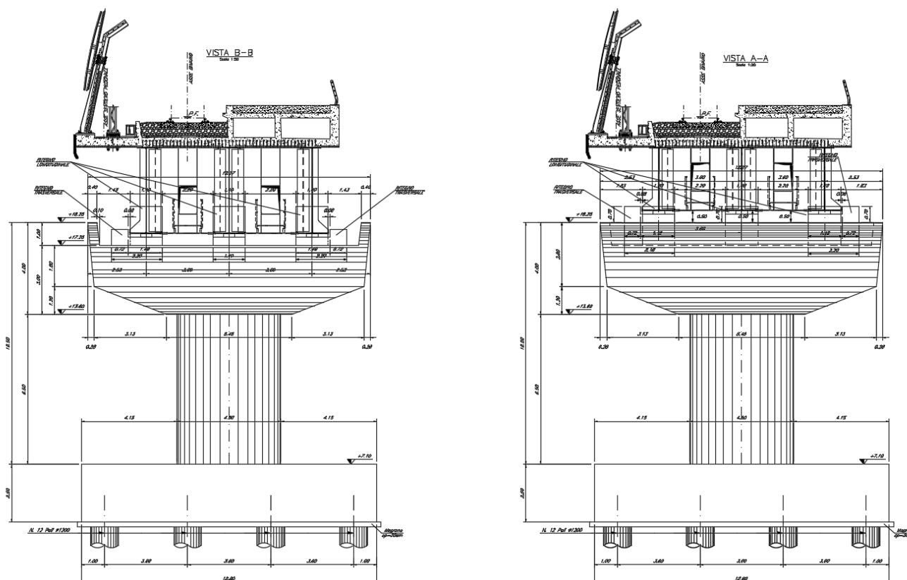
Figura 5 – prospetti pila
