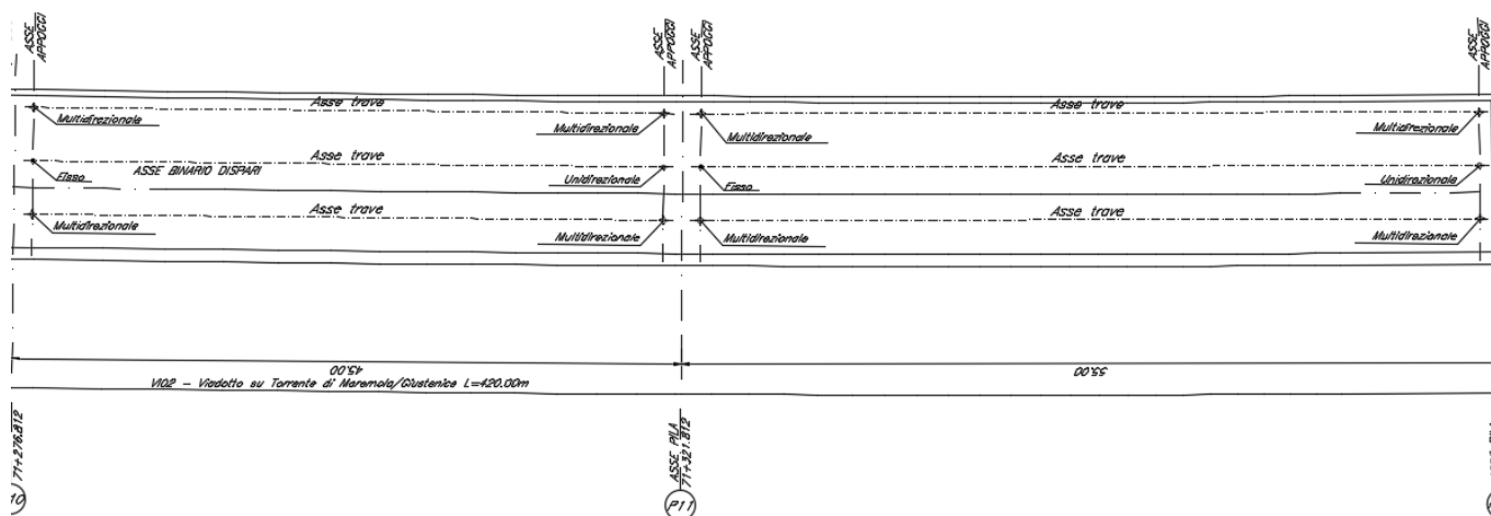
Figura 1 -schema appoggi impalcati convergenti sulla pila.
