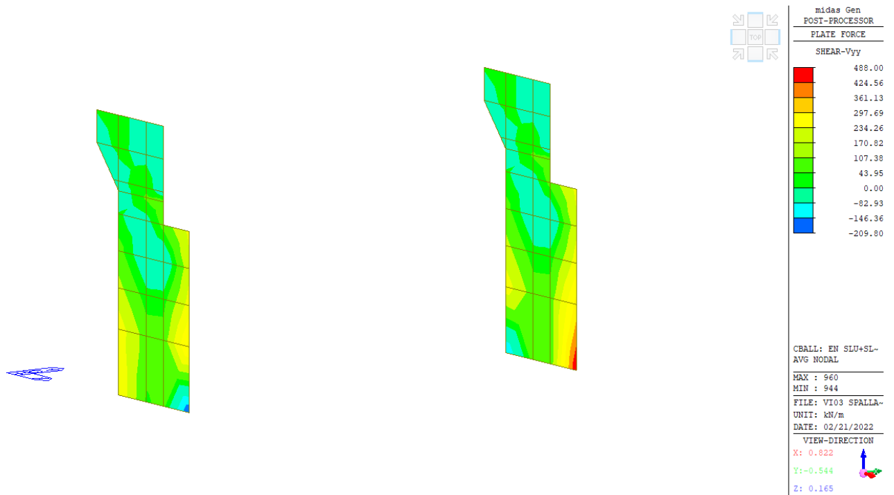
Inviluppo azione di taglio in direzione Y - SLU+ SLV
