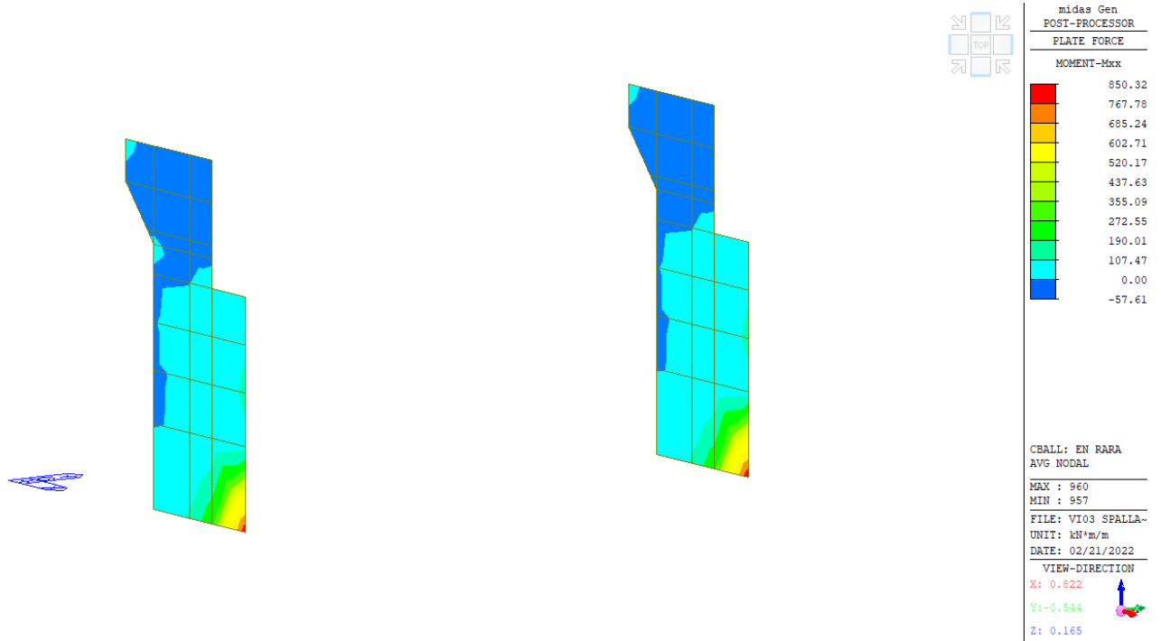
Inviluppo momento flettente in direzione X – SLE RARA
