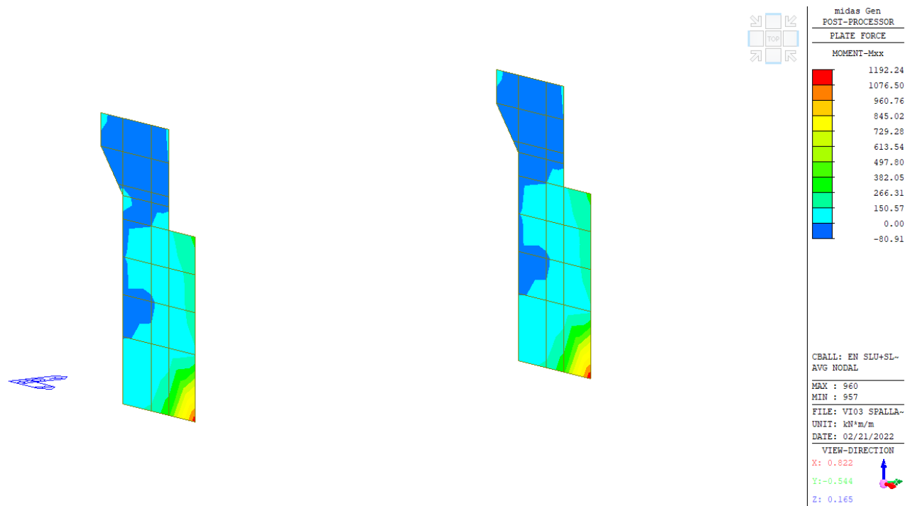
Involuppo momento flettente in direzione X - SLU+ SLV
