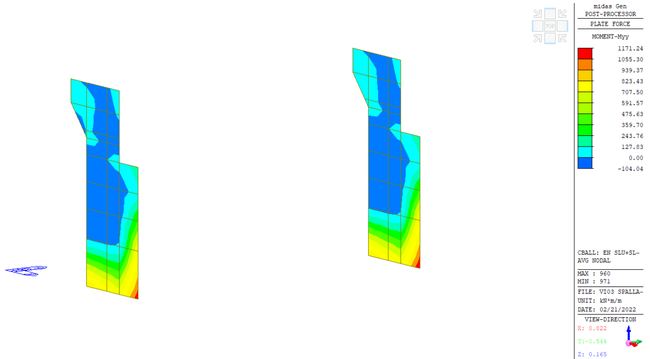
Inviluppo momento flettente in direzione Y – SLU+ SLV
