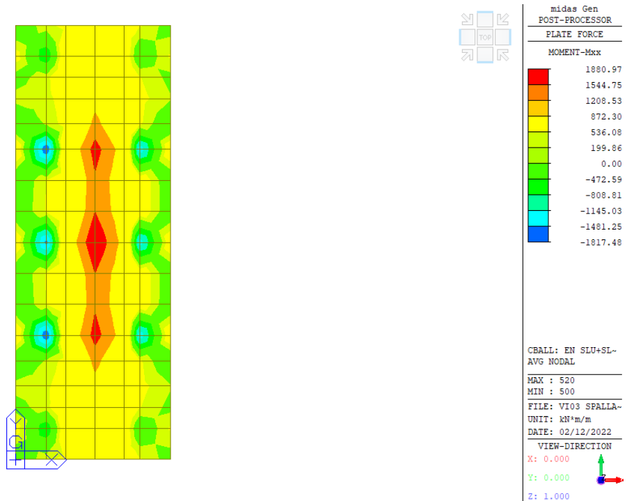
Inviluppo momento flettente in direzione X – SLU + SLV
