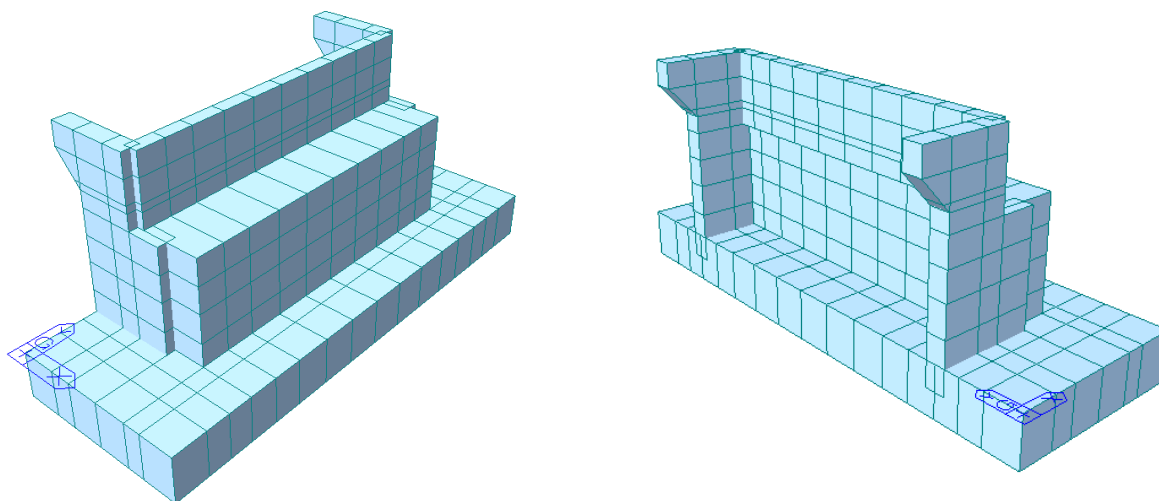
Figura 2 –Viste 3d del modello di calcolo spalla A (mobile)
