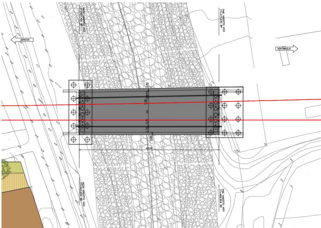
Figura 1: planimetria generale
