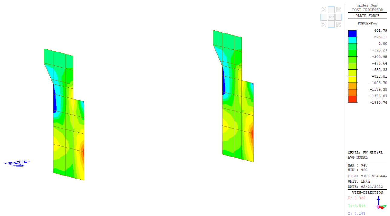
Inviluppo azione assiale verticale - SLU+ SLV
