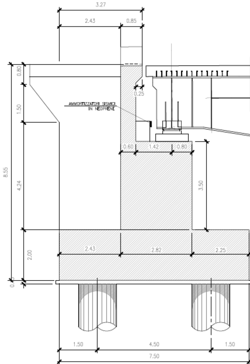
Figura 4: Spalla A
