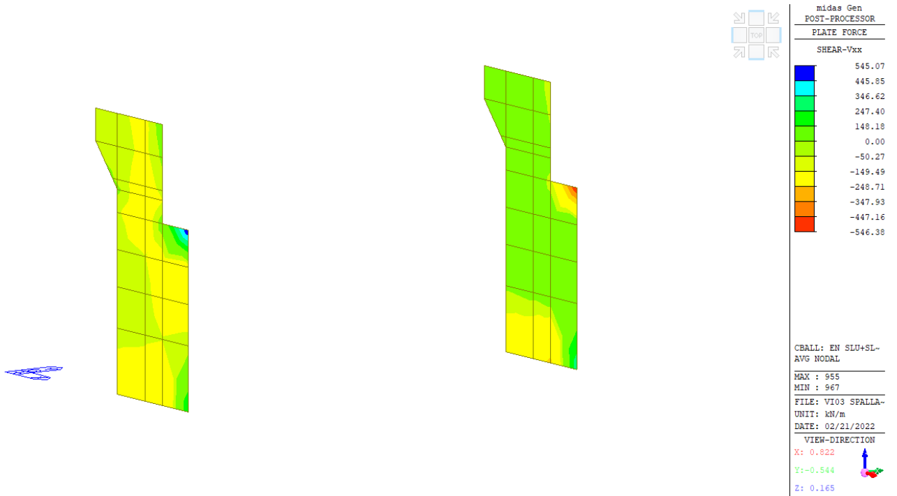
Inviluppo azione di taglio in direzione X - SLU+ SLV
