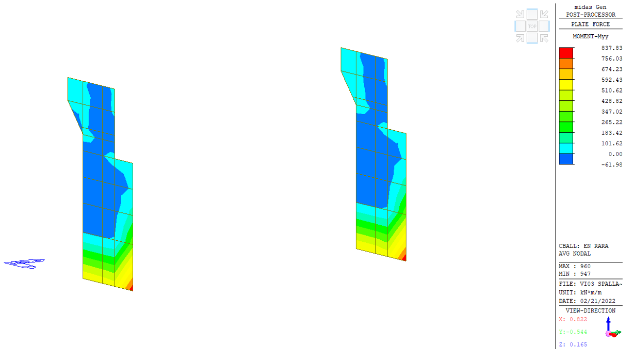
Inviluppo momento flettente in direzione Y – SLE RARA
