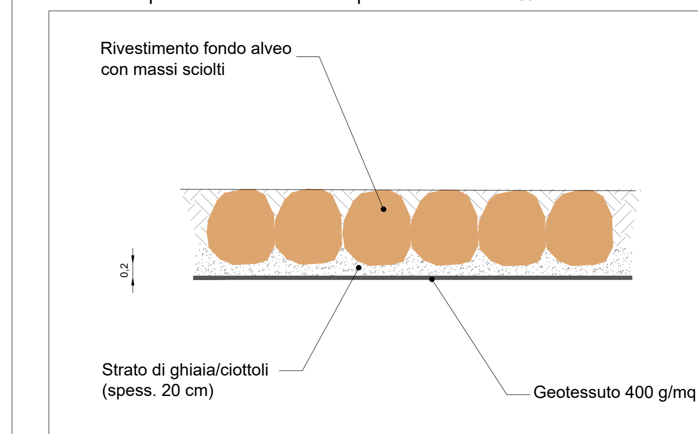
Particolare posa dei massi sciolti di protezione - scala 1:50
