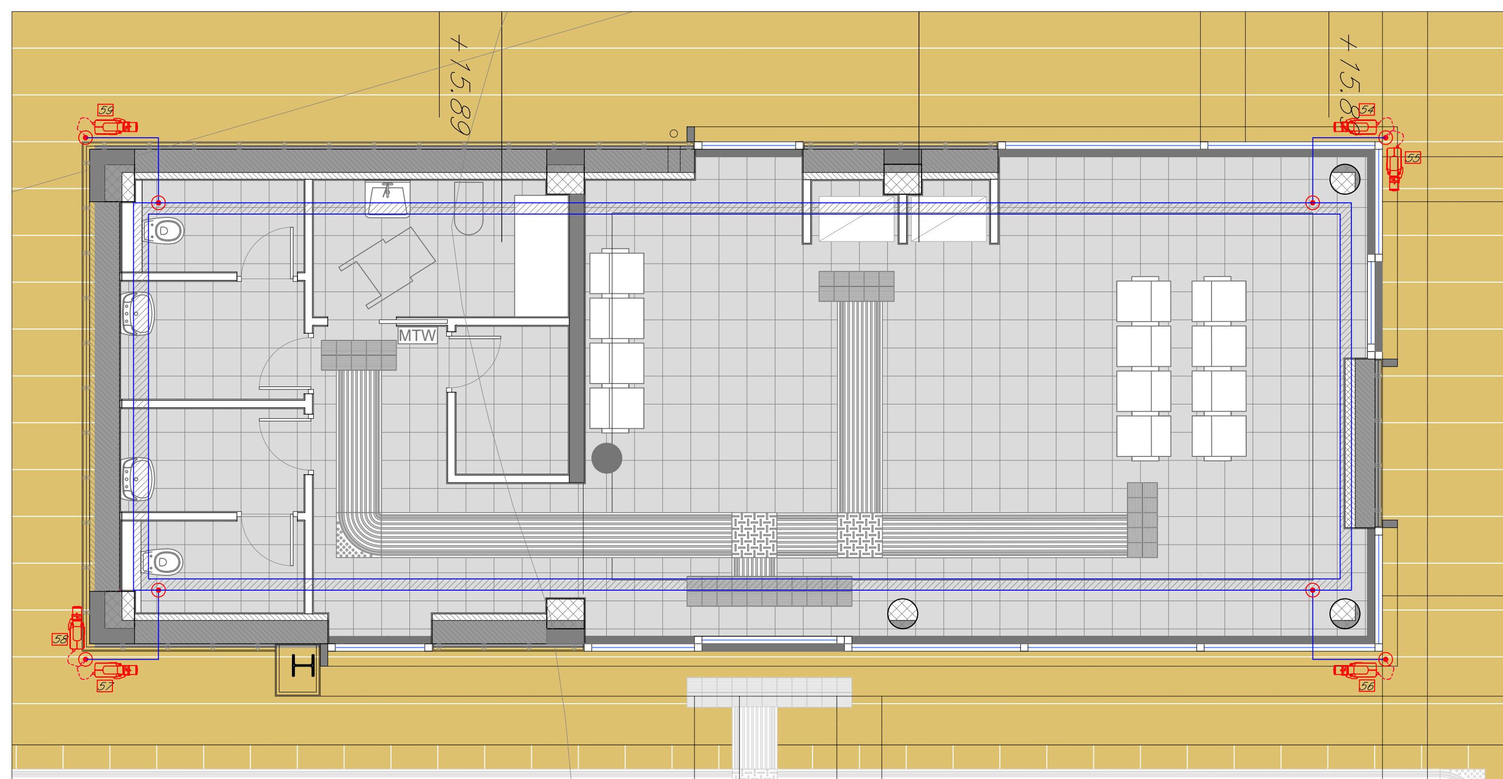
F.V. - PIANO TERRA - PIANTA AMBIENTE
