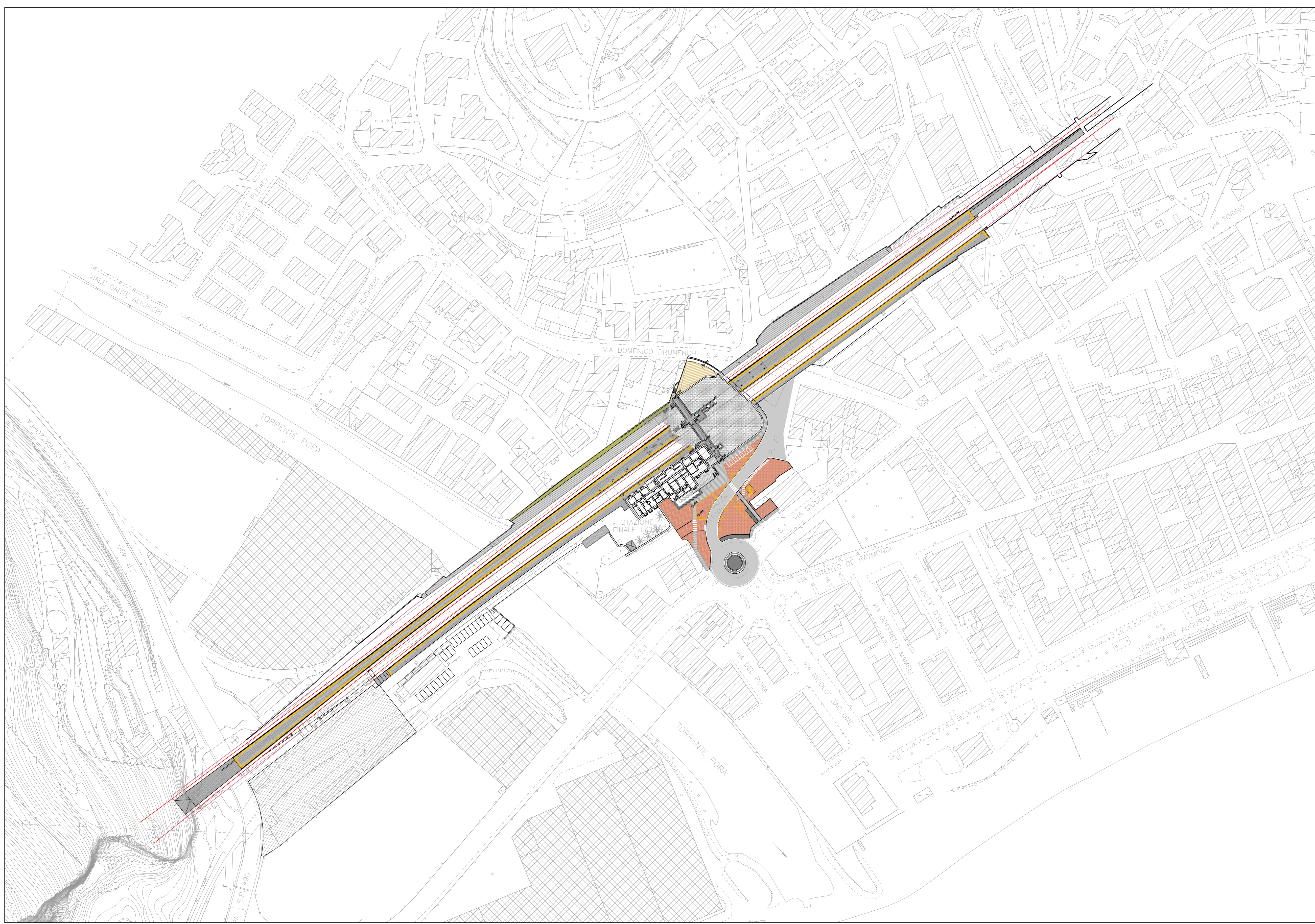
PIANTA CHIAVE - SCALA 1:1000
