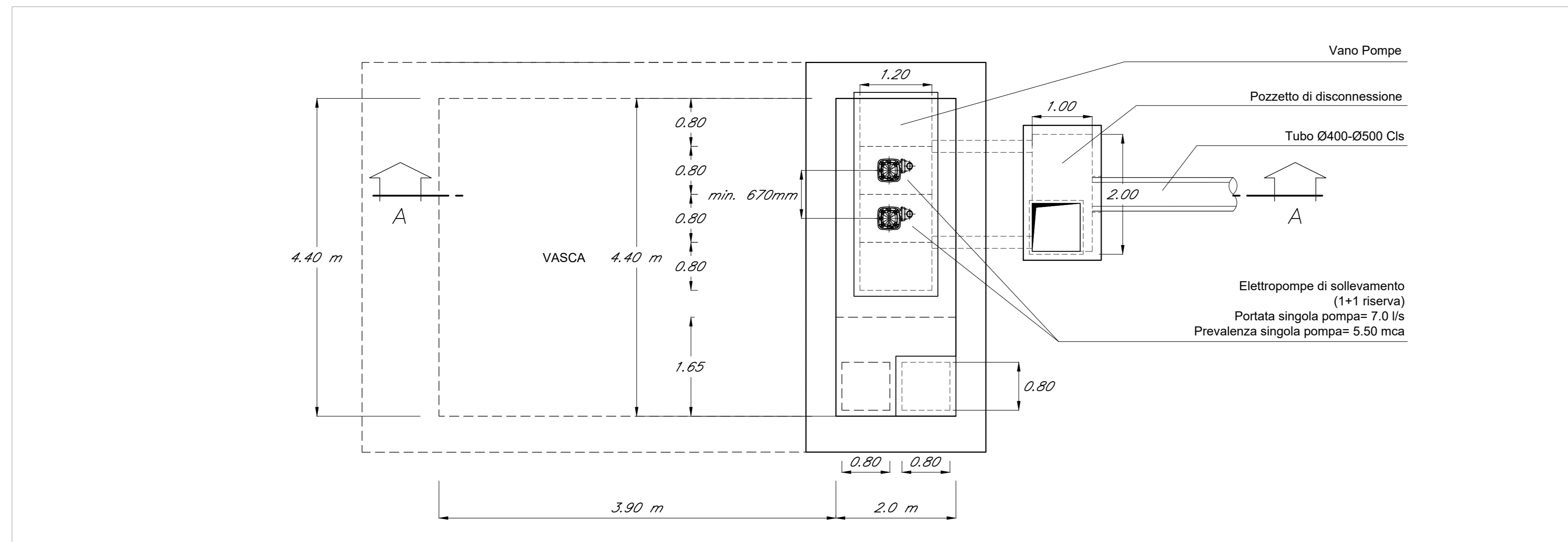
PIANTA - Scala 1:50
