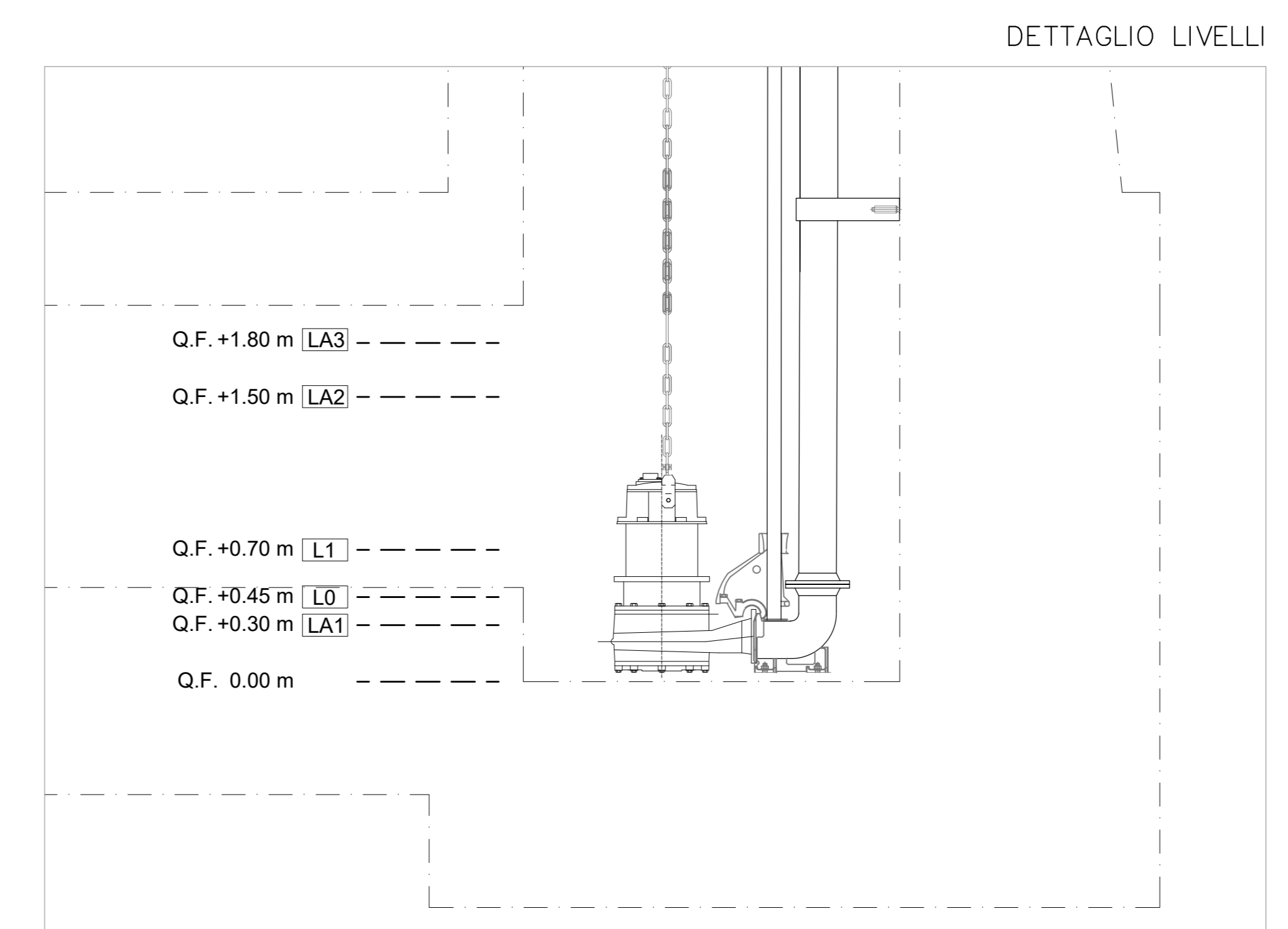
DETTAGLIO POMPA DI SOLLEVAMENTO
