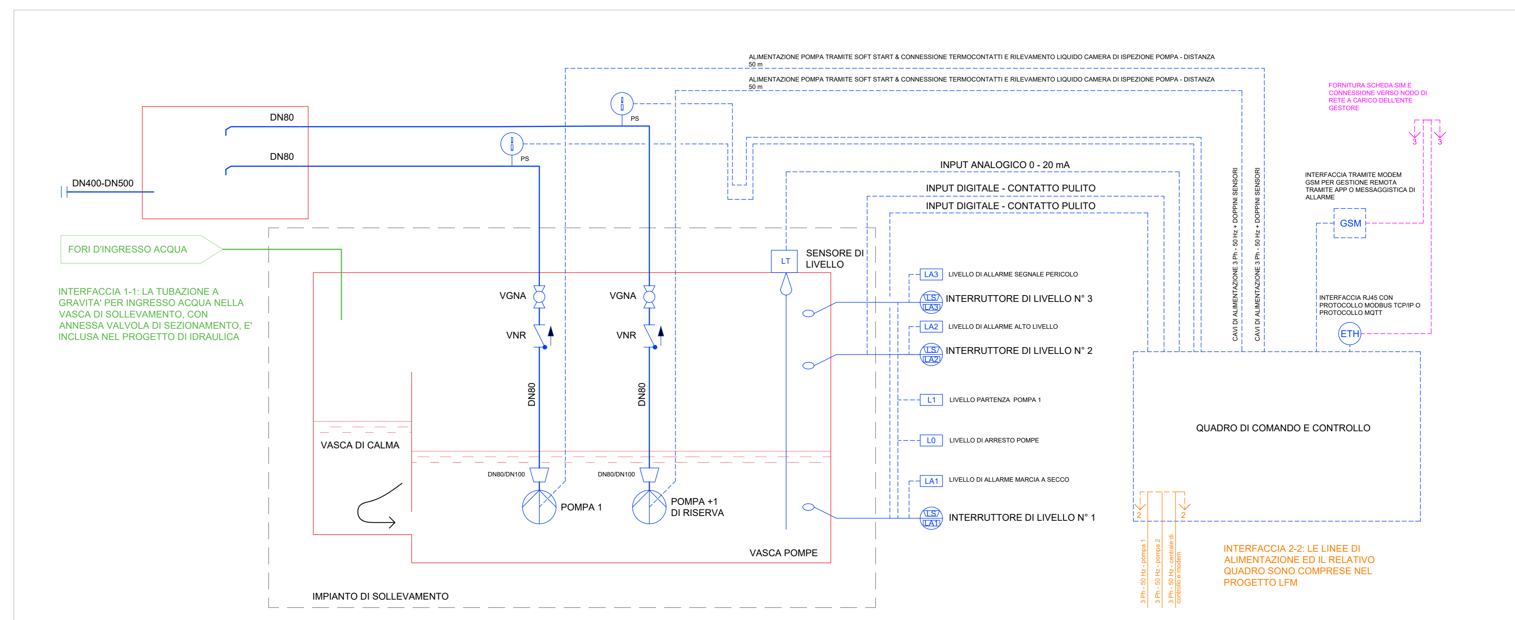
SCHEMA FUNZIONALE
