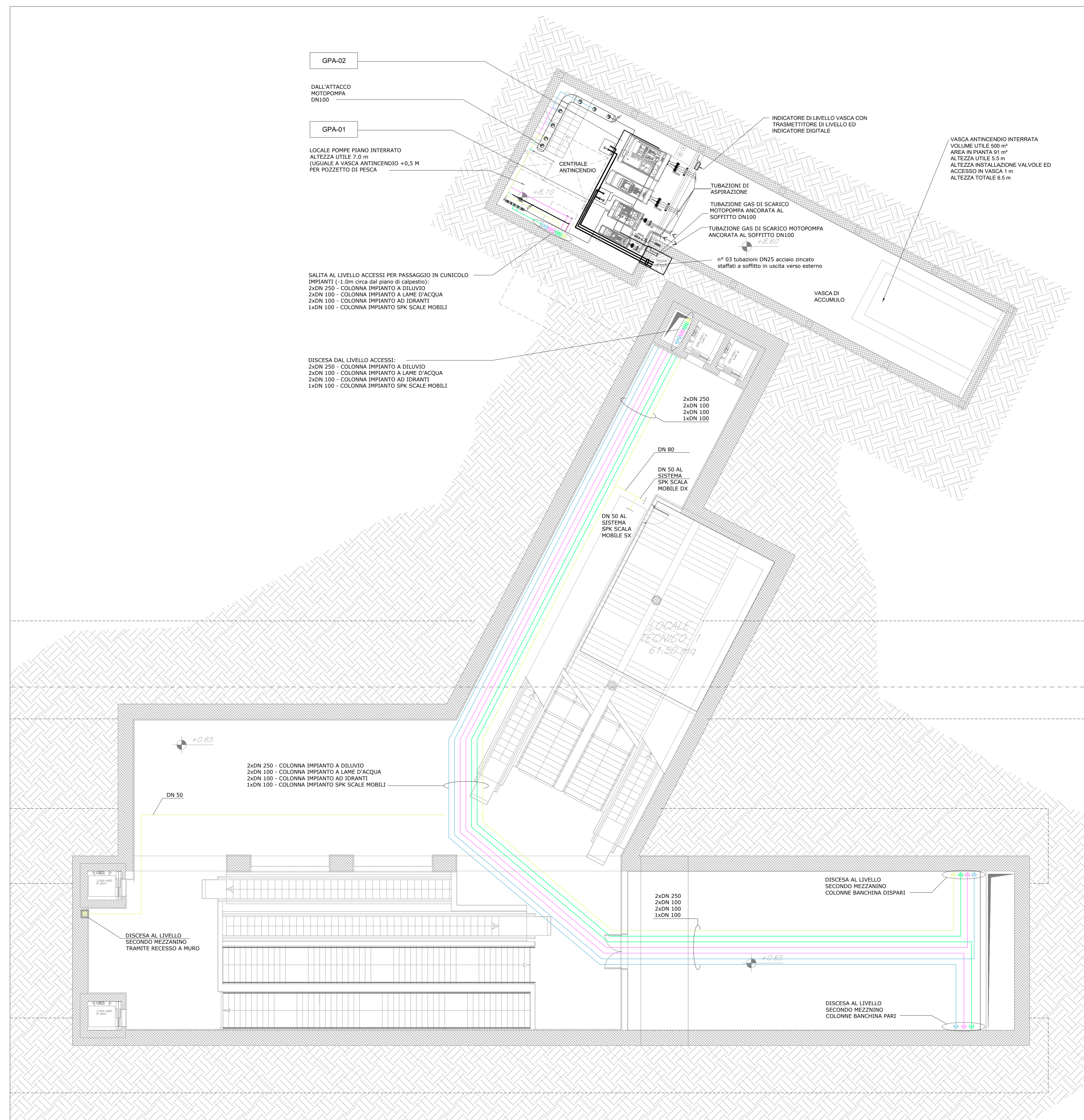
F.V. - PIANTA LIVELLO PRIMO MEZZANINO - SCALA 1:100 - USCITA GASTALDI
