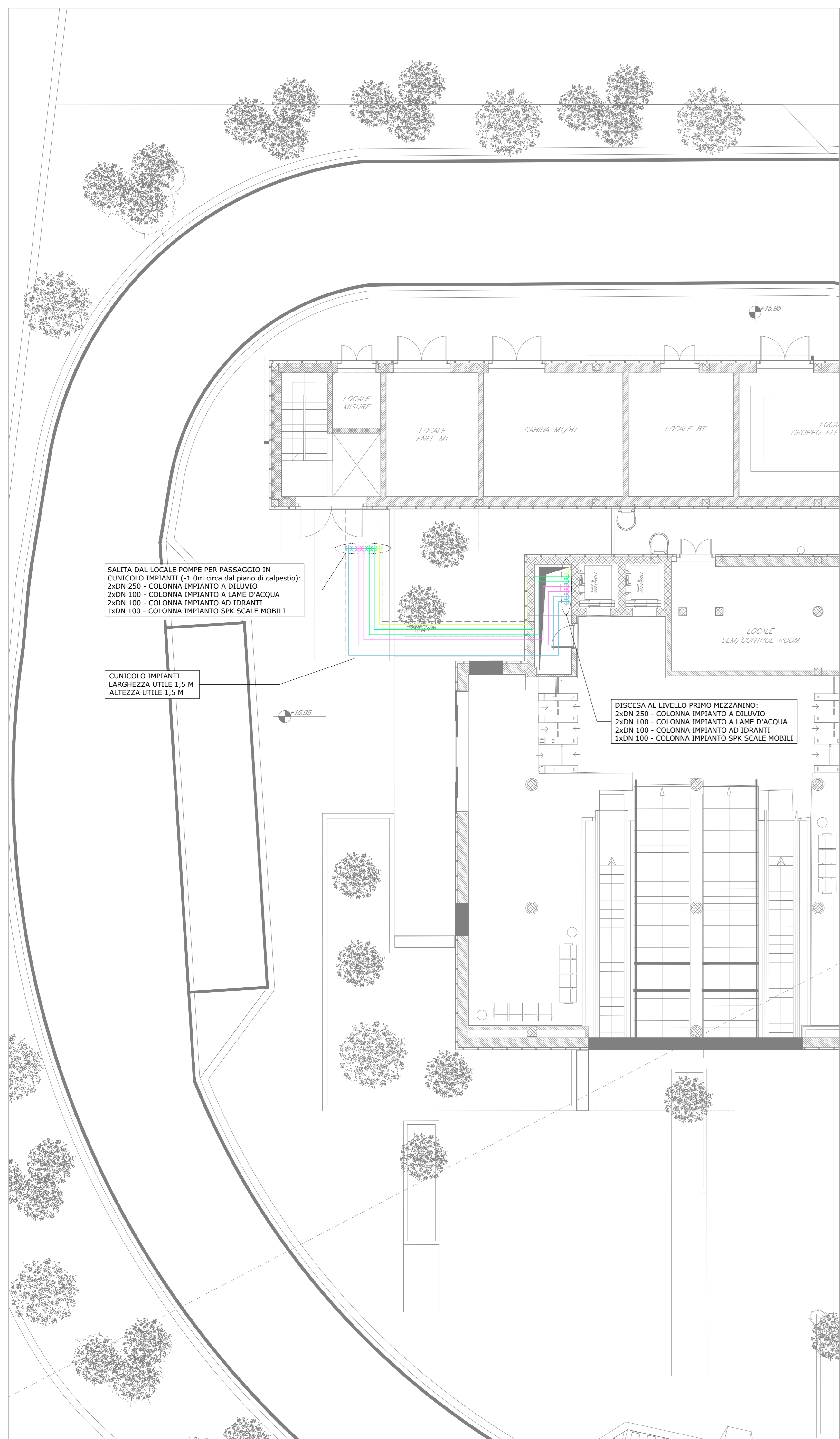
F.V. - PIANTA LIVELLO ACCESSI - SCALA 1:100 - USCITA GASTALDI
