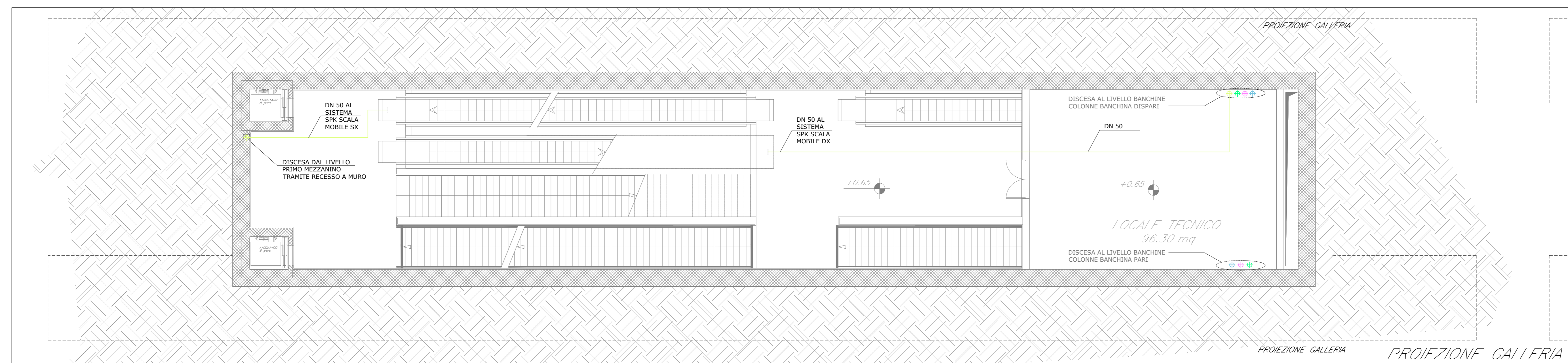
F.V. - PIANTA LIVELLO SECONDO MEZZANINO - SCALA 1:100 - USCITA GASTALDI
