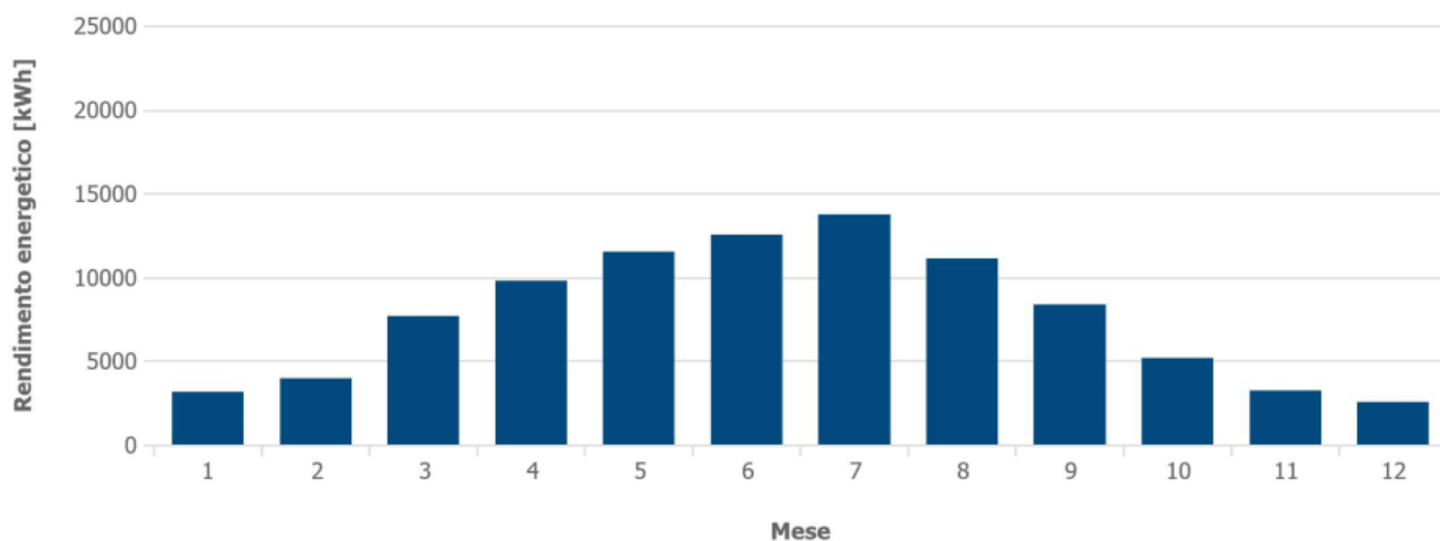
Figura 3 – Rendimento energetico mensile del Generatore FV
