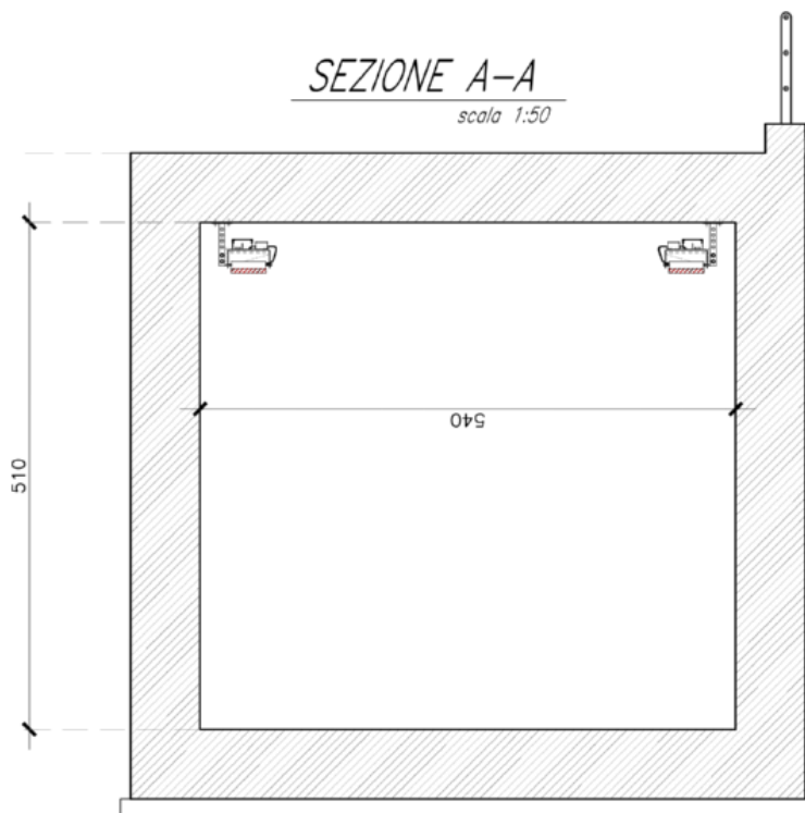
Figura 3 - Montaggio proiettori in sezione
