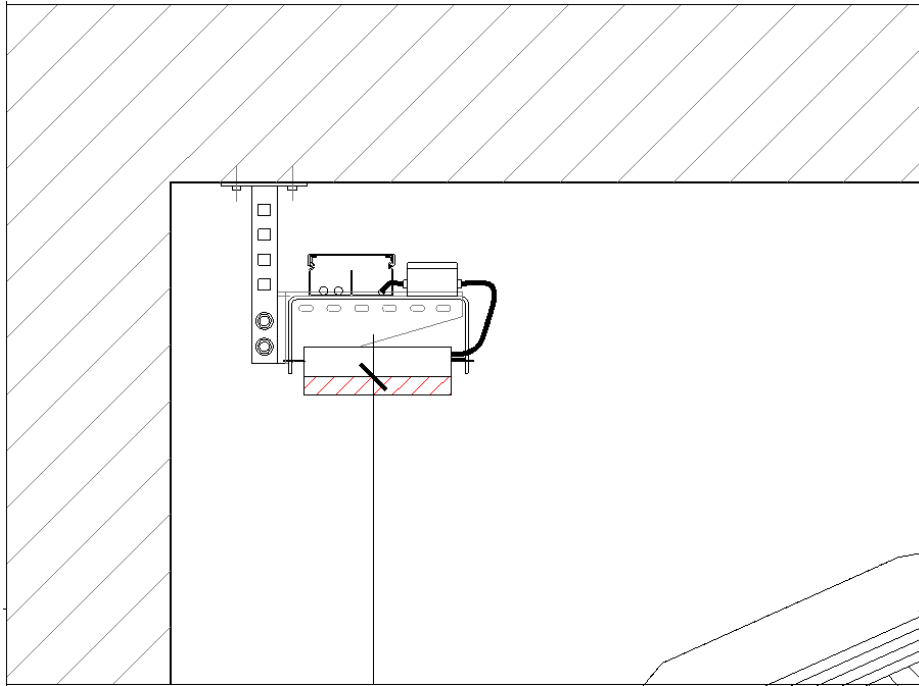
Figura 4 - Dettaglio montaggio
