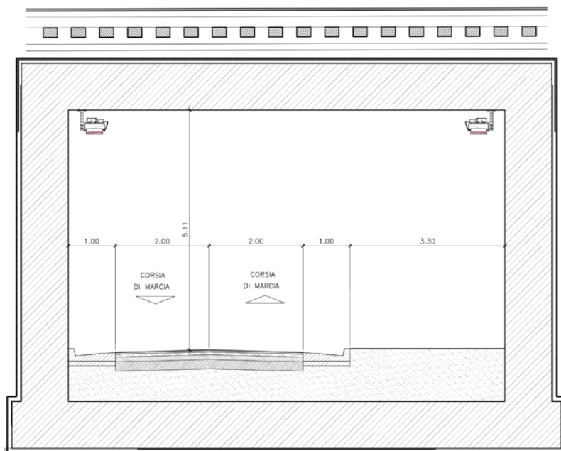
SEZIONE A-A
