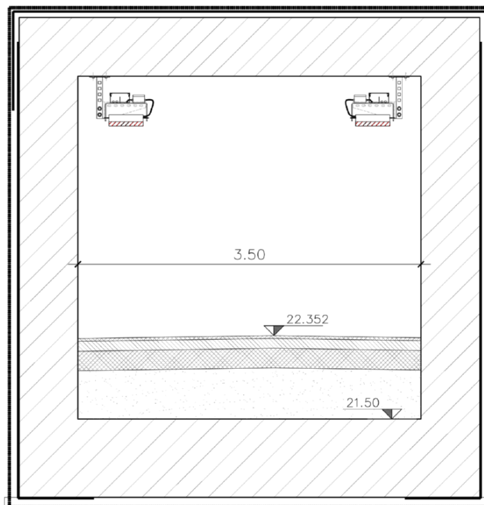
Figura 3 - Montaggio proiettori in sezione
