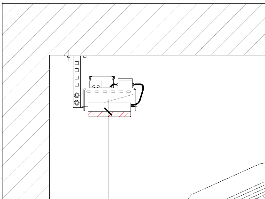
Figura 3 - Dettaglio montaggio
