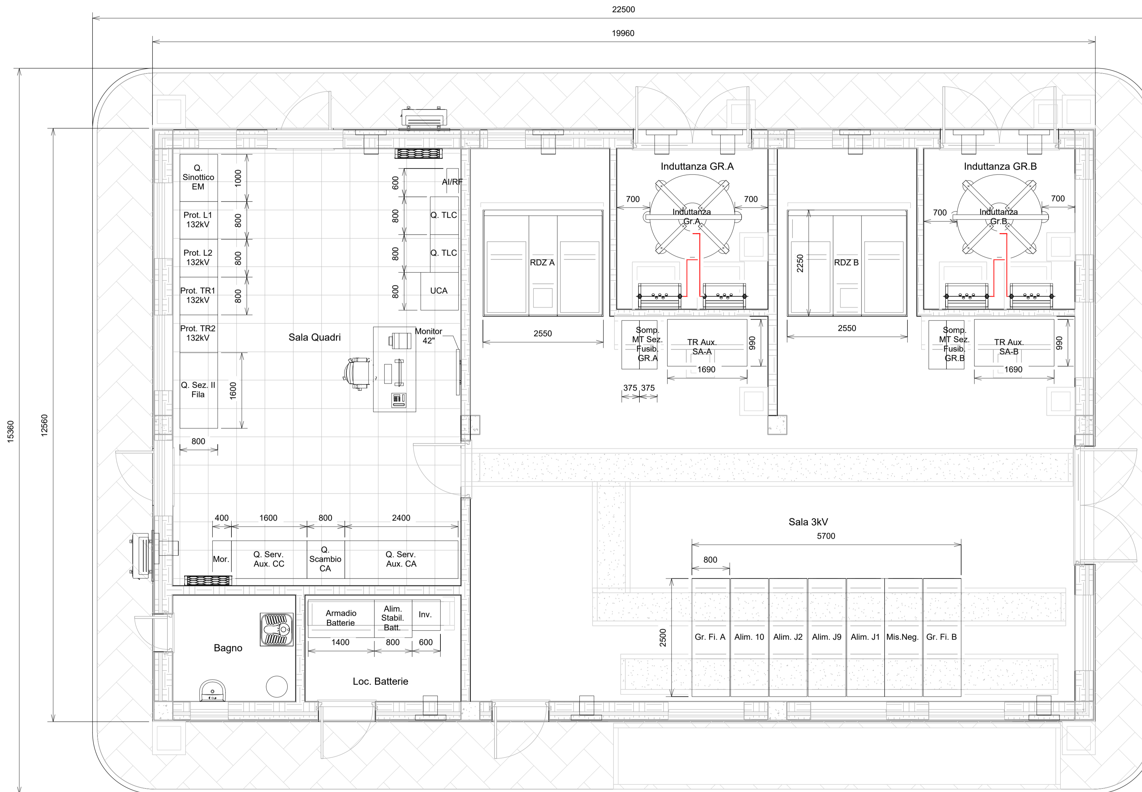
1 Disposizione apparecchiature (Layout) 1 : 50
