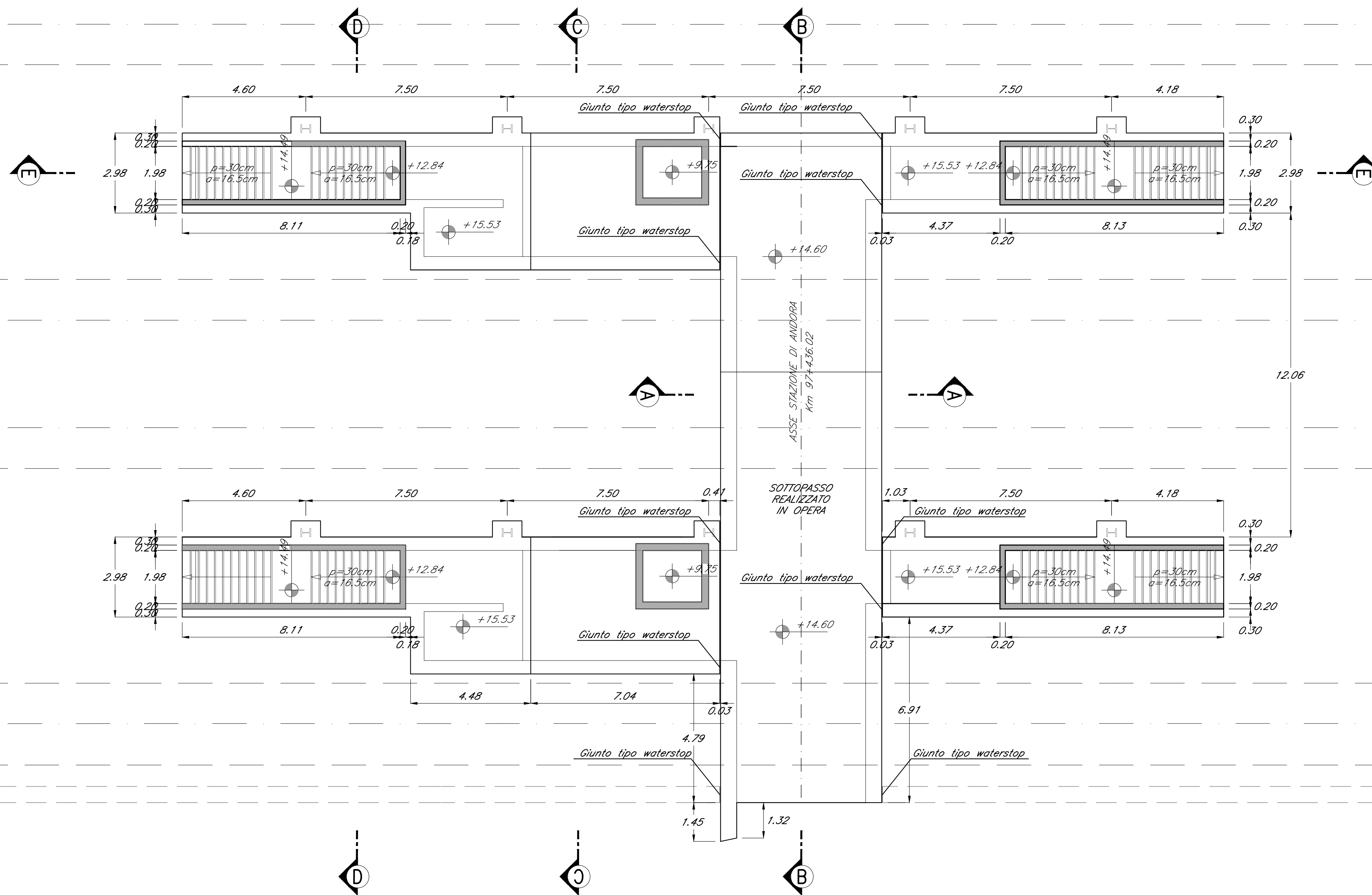
GG SEZIONE G-G scala 1:100
