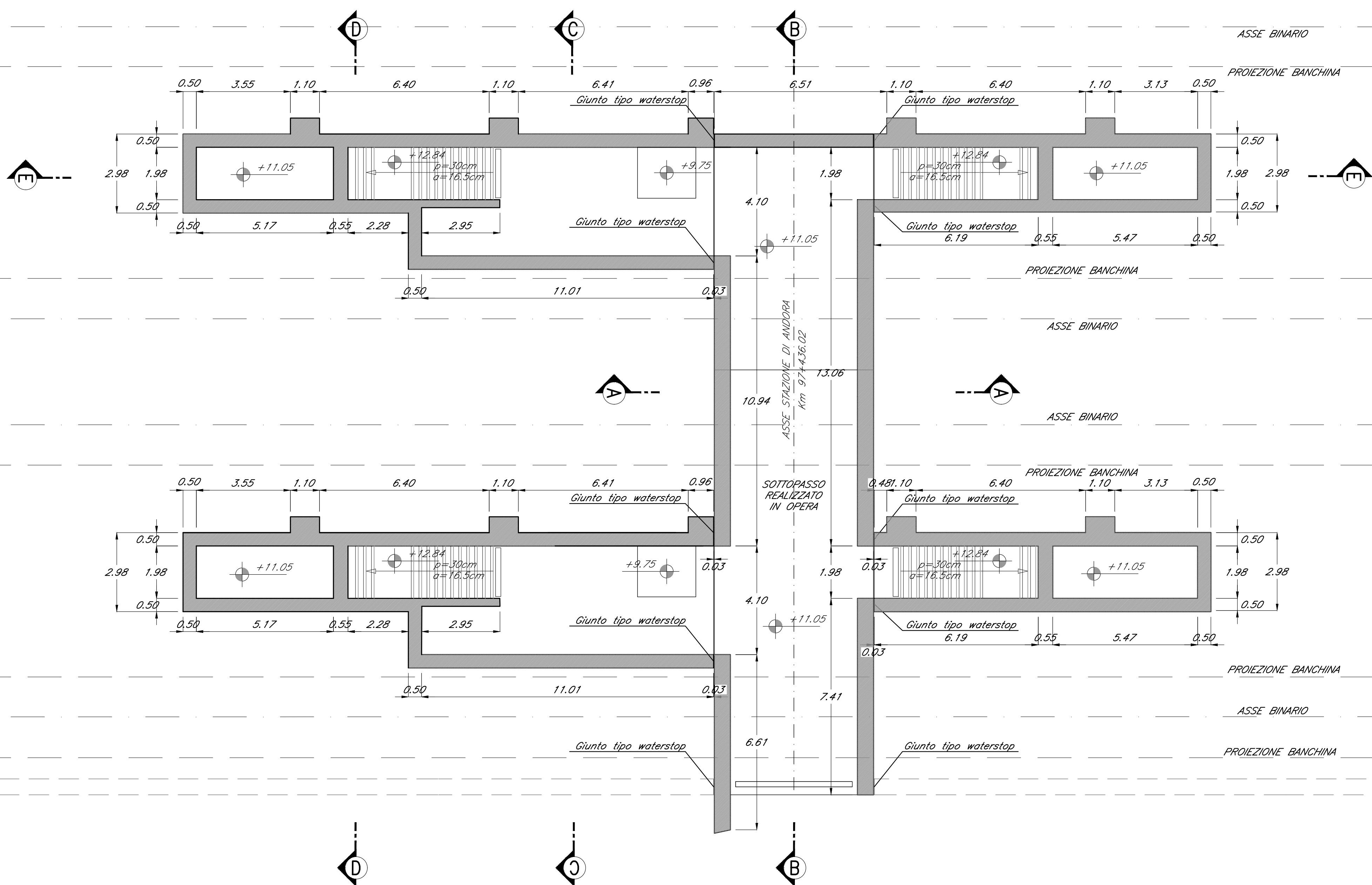
FF SEZIONE FF scala 1:100
