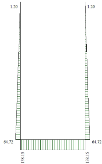
Figura 26 – Inviluppo diagramma sforzo normale SLE
