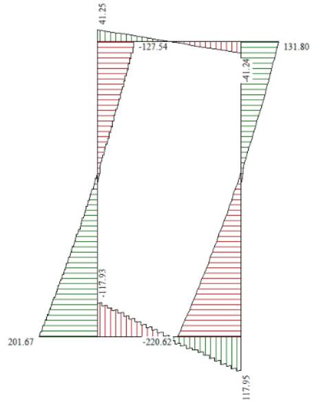
Figura 13 – Involuppo diagramma del taglio SLU
