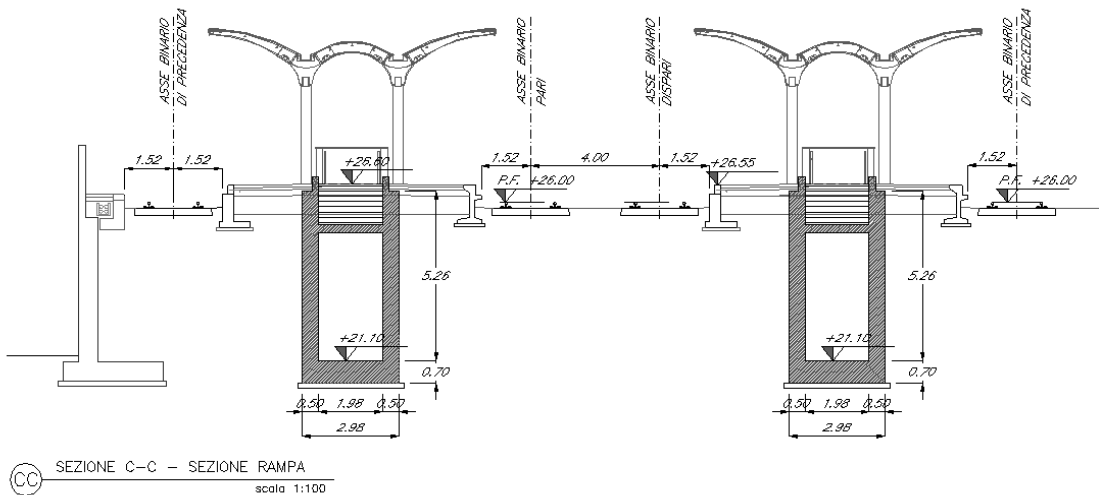
Figura 3 – sezione trasversale
