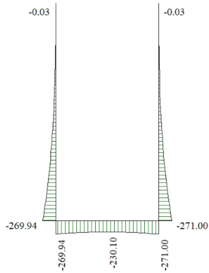
Figura 24- Involuppo momenti flettenti SLE
