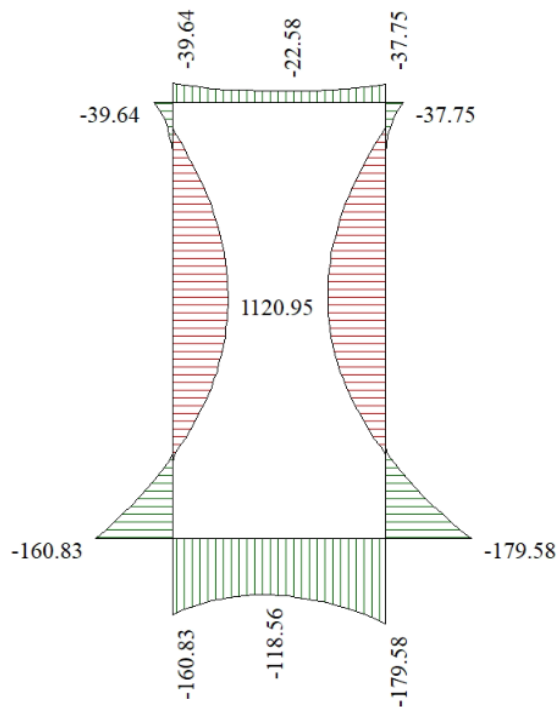
Figura 12 – Inviluppo diagramma dei momenti flettenti SLU
