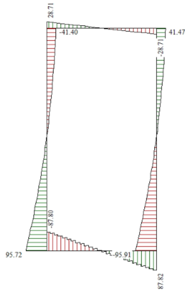
Figura 17 – Inviluppo diagramma del taglio SLE
