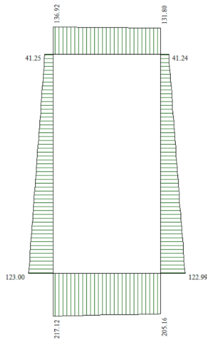
Figura 14 – involuppo diagramma sforzo normale SLU
