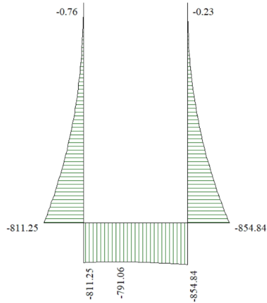
Figura 20 – Involuppo diagramma dei momenti flettenti SLU
