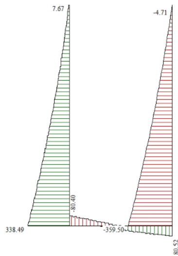
Figura 20 – Involuppo diagramma dei momenti flettenti SLU
