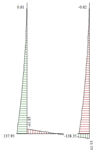
Figura 25 – Involuppo diagramma del taglio SLE
