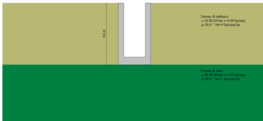
Figura 11 – Modello di calcolo scatolare sezione B
