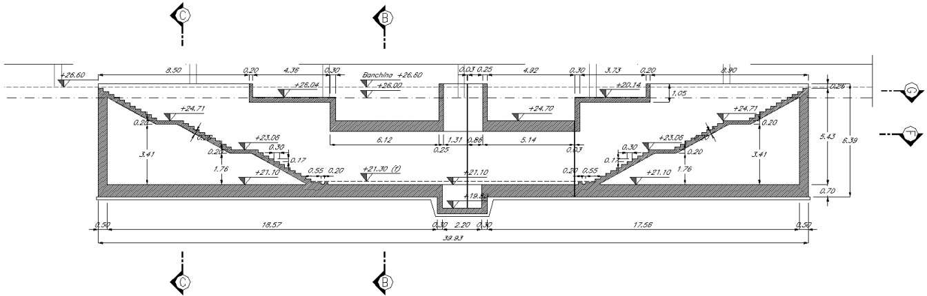
Figura 2 – Sezione longitudinale
