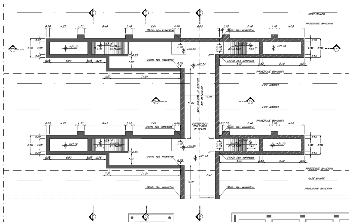
Figura 1 – Planimetria
