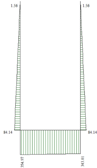
Figura 22 – inviluppo diagramma sforzo normale SLU
