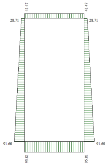
Figura 18 – Inviluppo diagramma sforzo normale SLE
