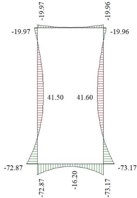
Figura 16- Inviluppo momenti flettenti SLE
