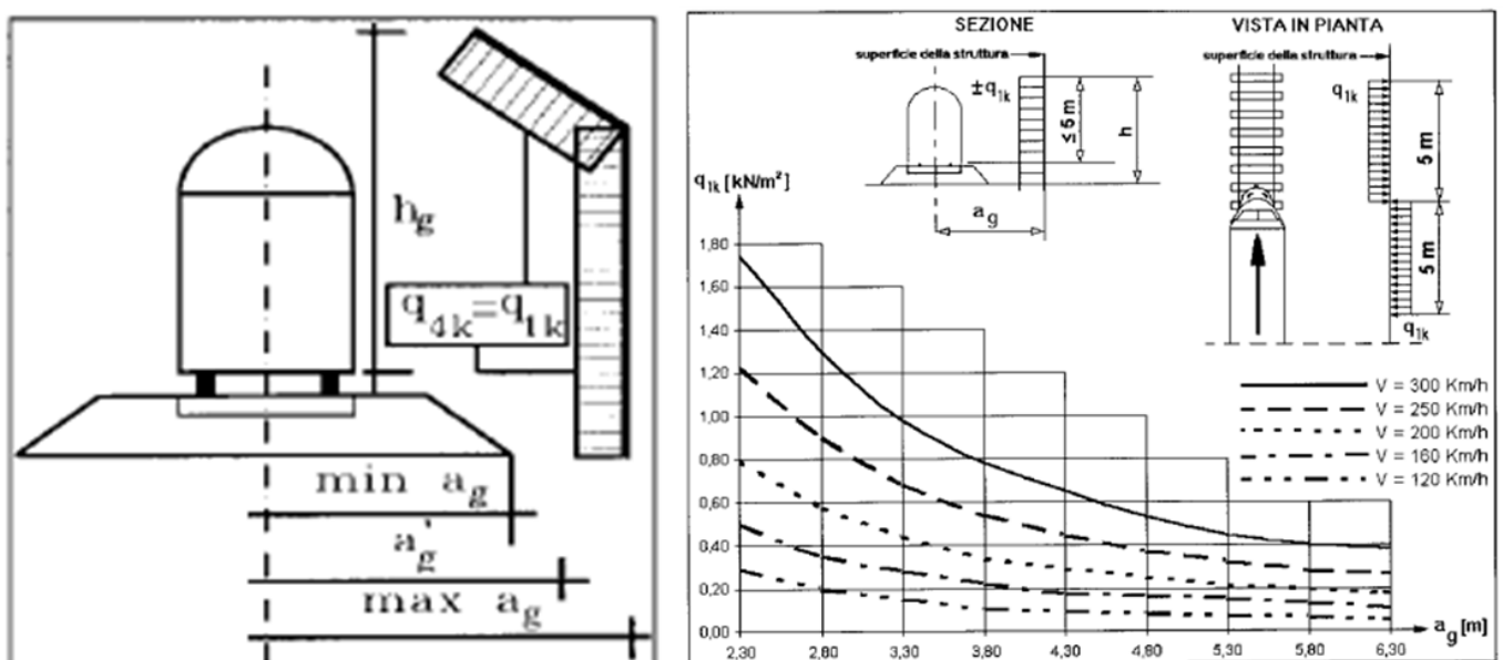
Figura 2- Grafico per la definizione della distanza \min - \max a_g , e valori caratteristici delle azioni q_{1k} su superfici verticali e parallele al binario
