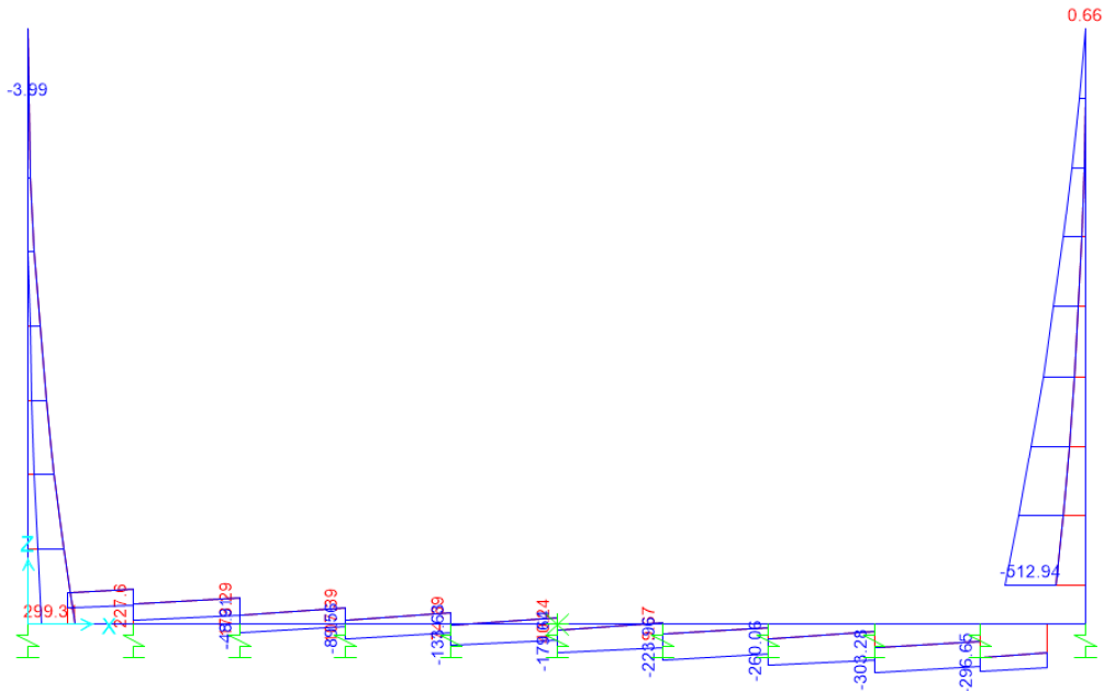
Figura 12: Taglio – Involuppo SLU (kN)
