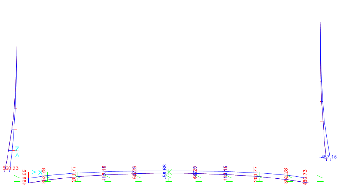
Figura 15: Momento flettente – Inviluppo SLE-Rara (KNm)
