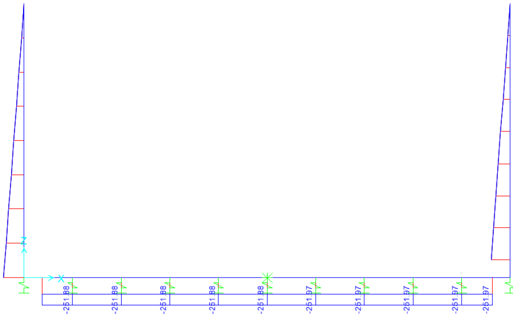
Figura 14: Sforzo normale – Inviluppo SLE Rara (kN)
