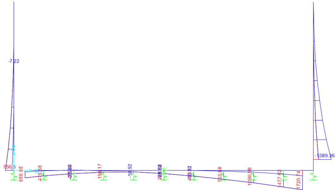
Figura 13: Momento flettente – Inviluppo SLU (kNm)
