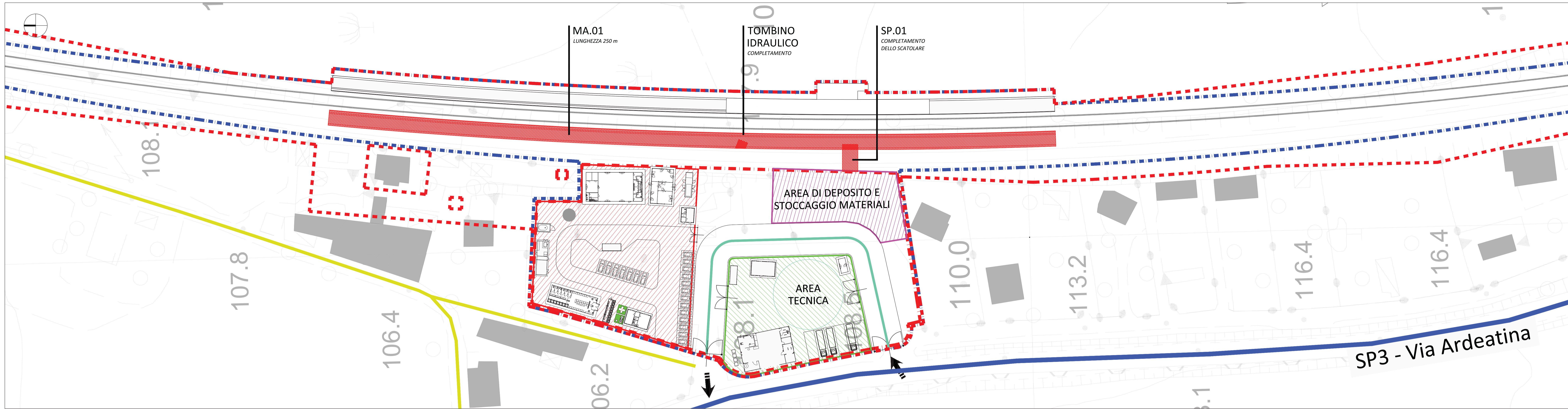
2 Macrofase 04.b - Realizzazione marciapiede pari 1:1000
