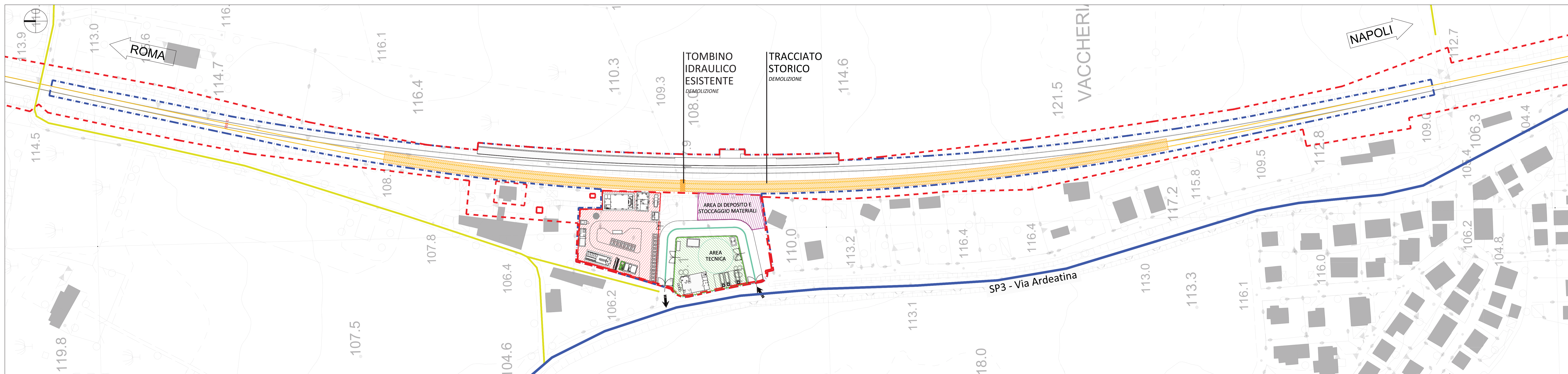
1 Macrofase 04.a - Opere di dismissione vecchio tracciato 1:1000
