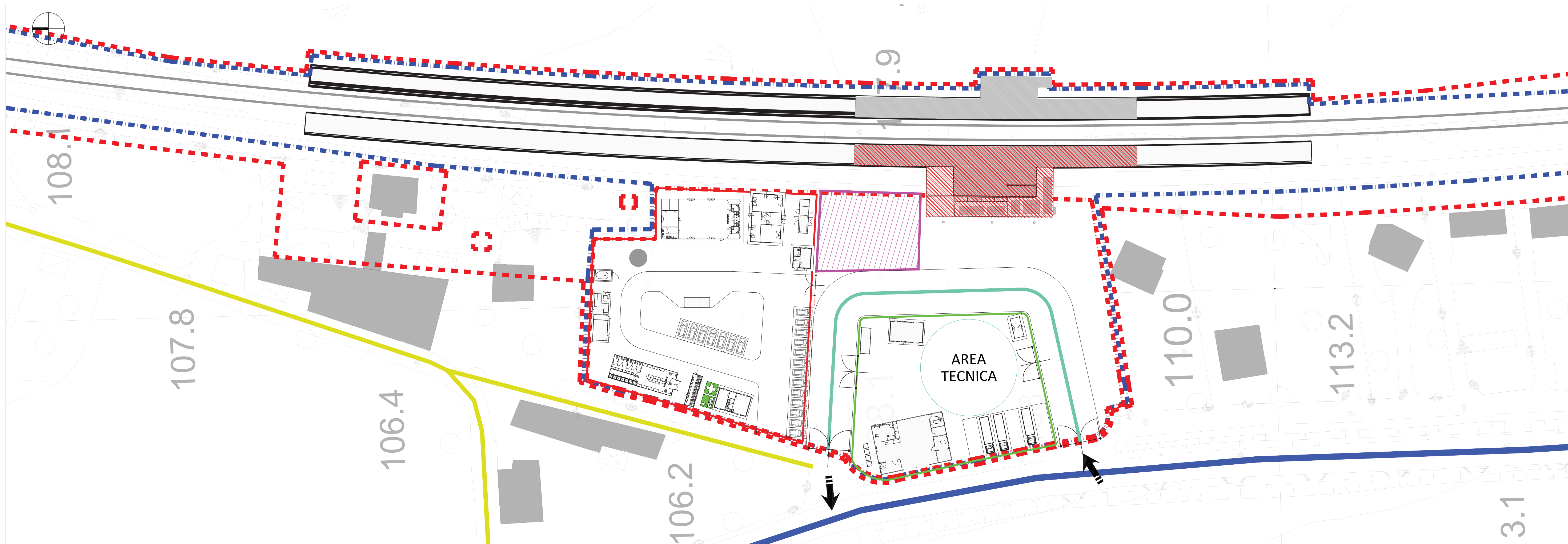
1 Macrofase 05.a - Realizzazione Fabbricato Viaggiatori e pensilina primo marciapiede 1 : 500
