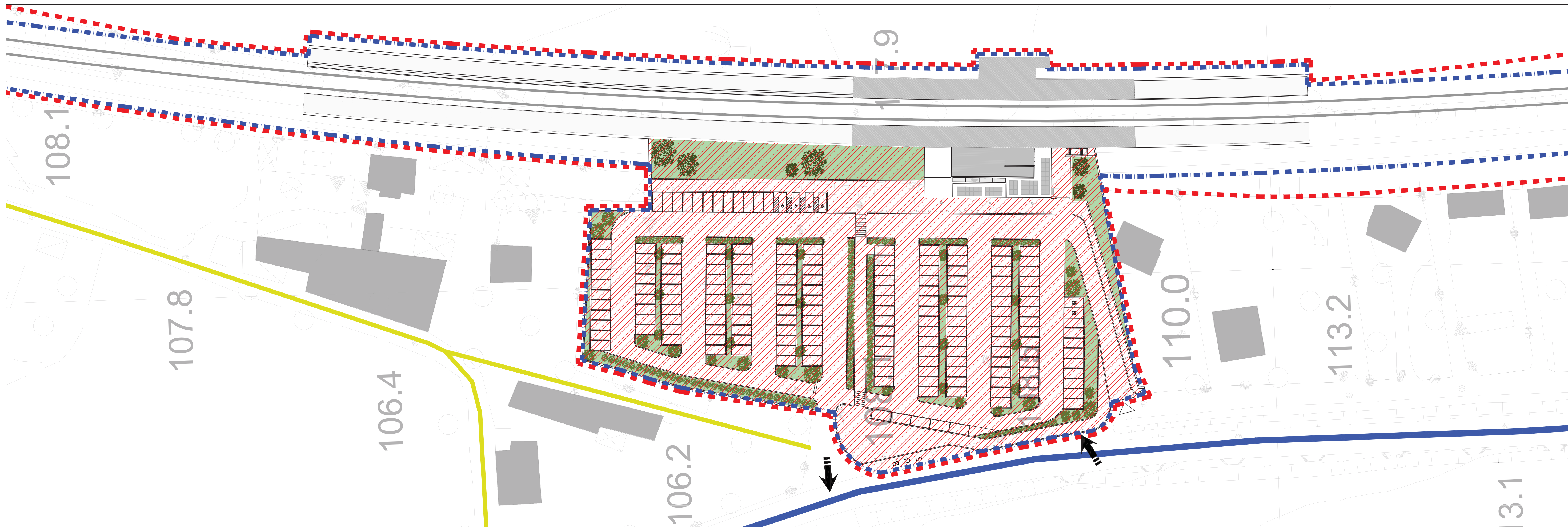
2 Macrofase 05.b - Realizzazione Piazzale di stazione 1 : 500
