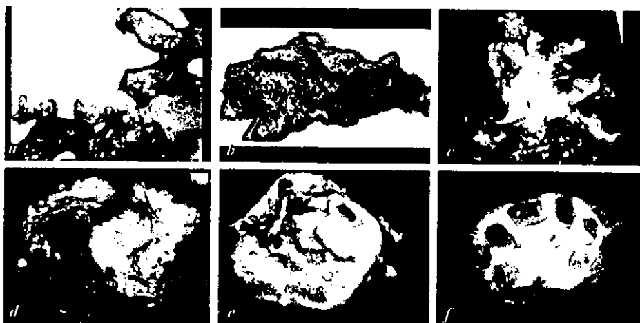
Alcune specie di Spugne della biocenosi dei Coralli Profondi: (a) Spongosorites sp.; (b) Pocillastra compressa ; (c) Thrombus abyssis ; (d) Pachastrella monilifera ; (e) Erylus papulifer , (f) Spiroxya levispira (da Mastrototaro et al., 2010).
