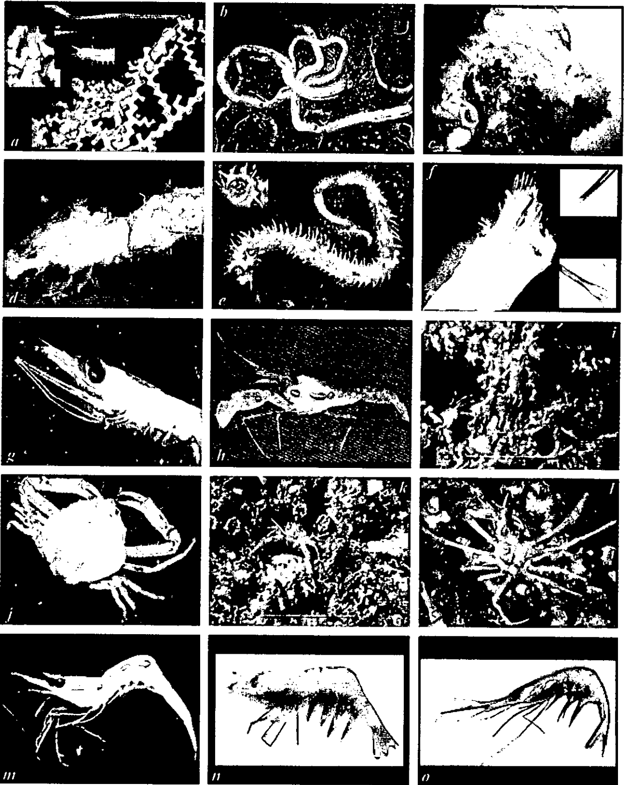
Alcune specie di Annelidi e Crostacei della biocenosi dei Coralli Profondi: (a) Eunice norvegica; (b) Metavermilia multicristata; (c) Vermiliopsis monodiscus; (d) Serpula vermicularis; (e) Vermiliopsis iseliasoni; (f) Phalacrostemma sp.; (g) Stylocheiron suhmii; (h) Alpheus platydactylus; (i) Bathynectes maravigna; (j) Ebalia nux; (k) Munida sp.; (l): Rochinia rissoana; (m) Pandalina profunda; (n) Plesionika acanthonotus; (o) Plesionika martia (da Mastrototaro et al., 2010).
