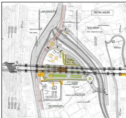
Figure 1 - Planimetria di progetto
