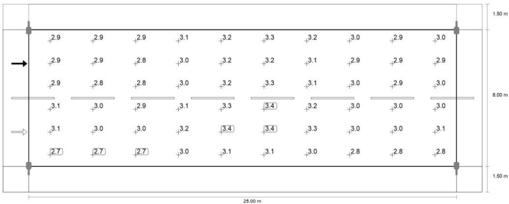
Osservatore 2: Luminanza per nuova installazione [ \text{cd/m}^2 ] (Raster dei valori)
