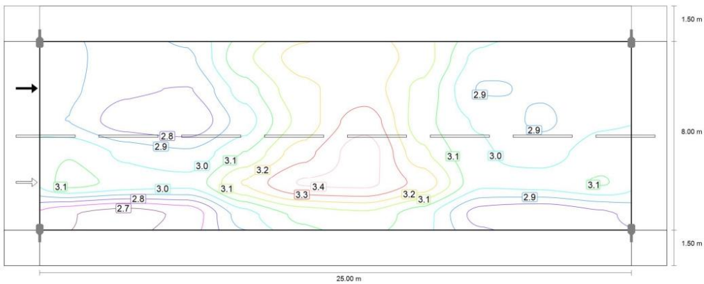
Osservatore 2: Luminanza per nuova installazione [ \text{cd/m}^2 ] (Curve isolux)
