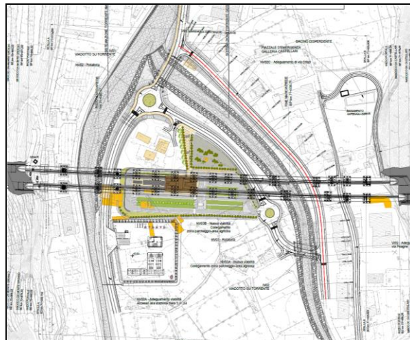
Figure 1-Planimetria di progetto
