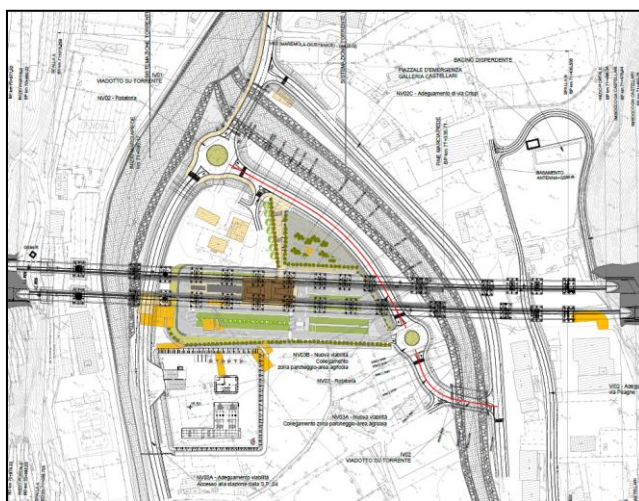
Figura 1 - Planimetria di progetto
