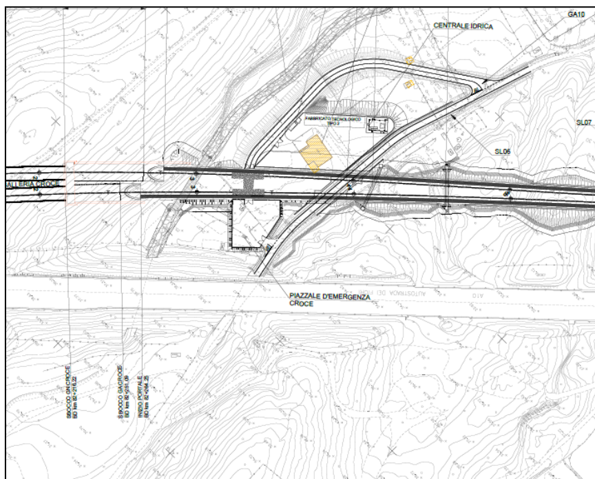
Figura 1 - Planimetria viabilità
