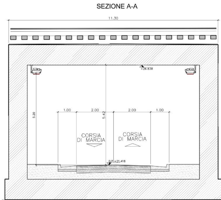
Figura 3 - Montaggio proiettori in sezione
